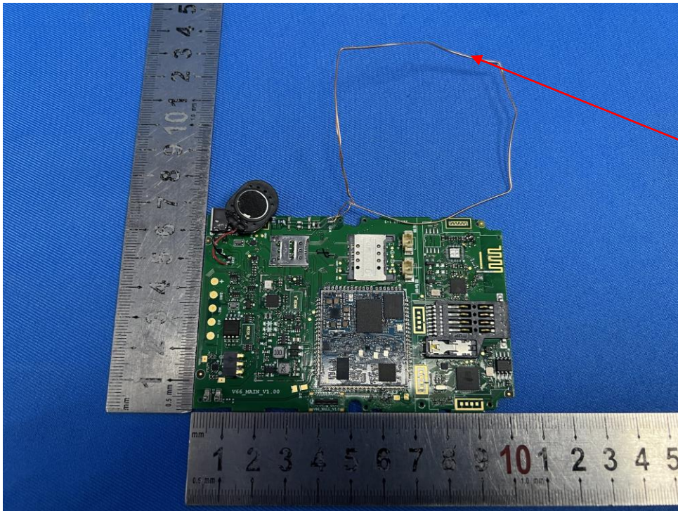
NFC Antenna
