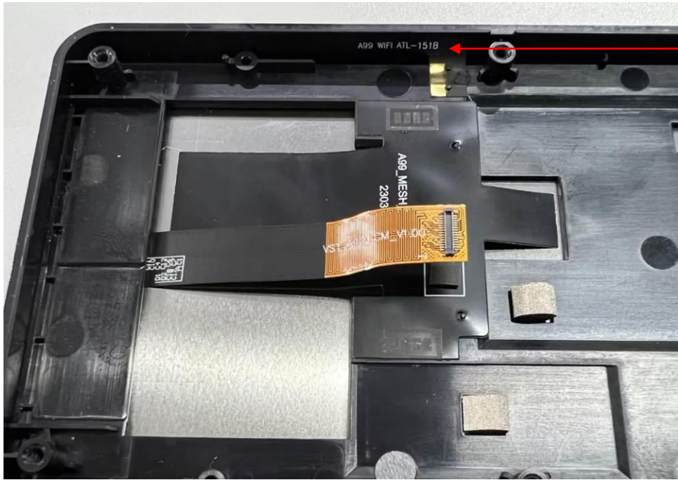
BT/WIFI antenna
