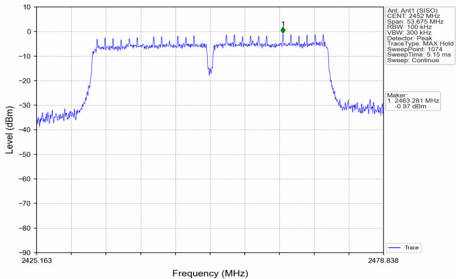
802.11n(HT40)_HCH_2452MHz_Ant1 (SISO)_NTNV
