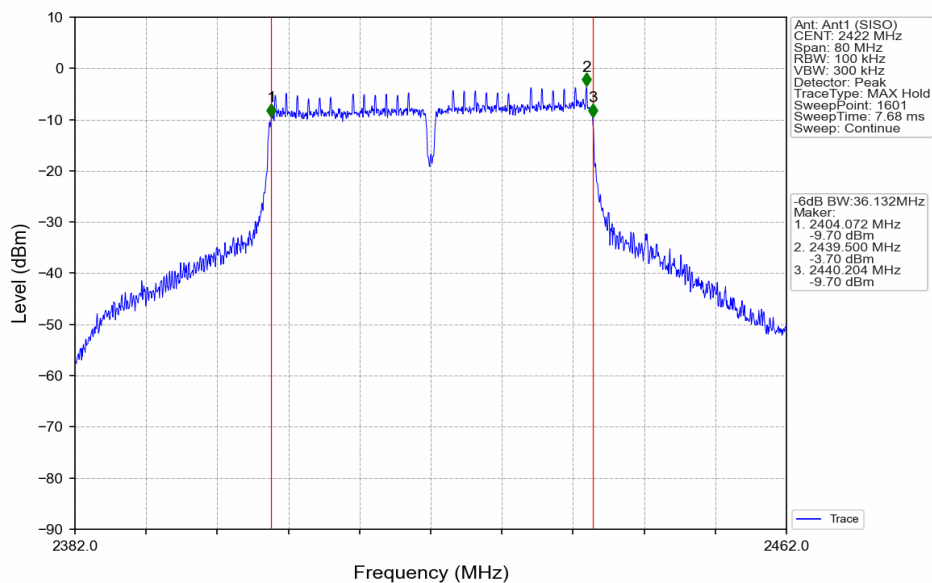
802.11n(HT40)_LCH_2422MHz_Ant1 (SISO)_NTNV
