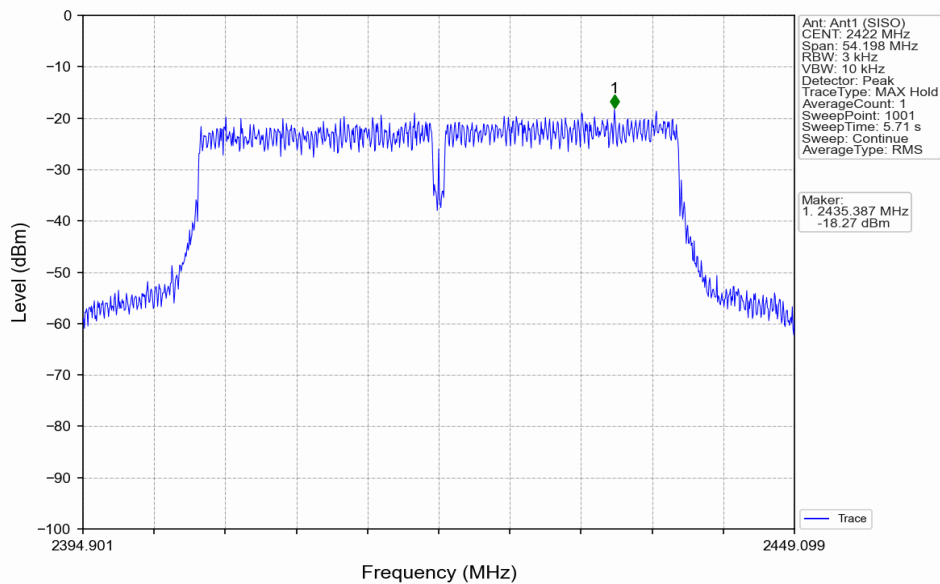
802.11n(HT40)_LCH_2422MHz_Ant1 (SISO)_NTNV
