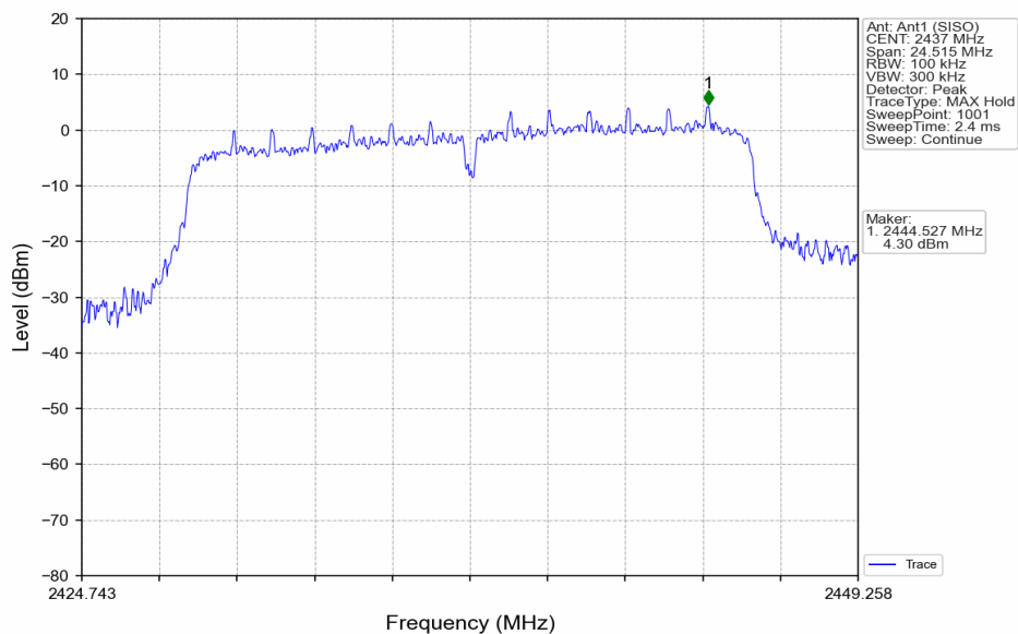
802.11n(HT20)_MCH_2437MHz_Ant1 (SISO)_NTNV
