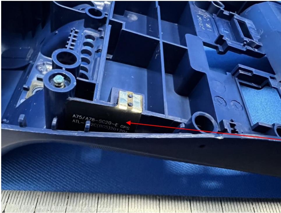
GPS Antenna
