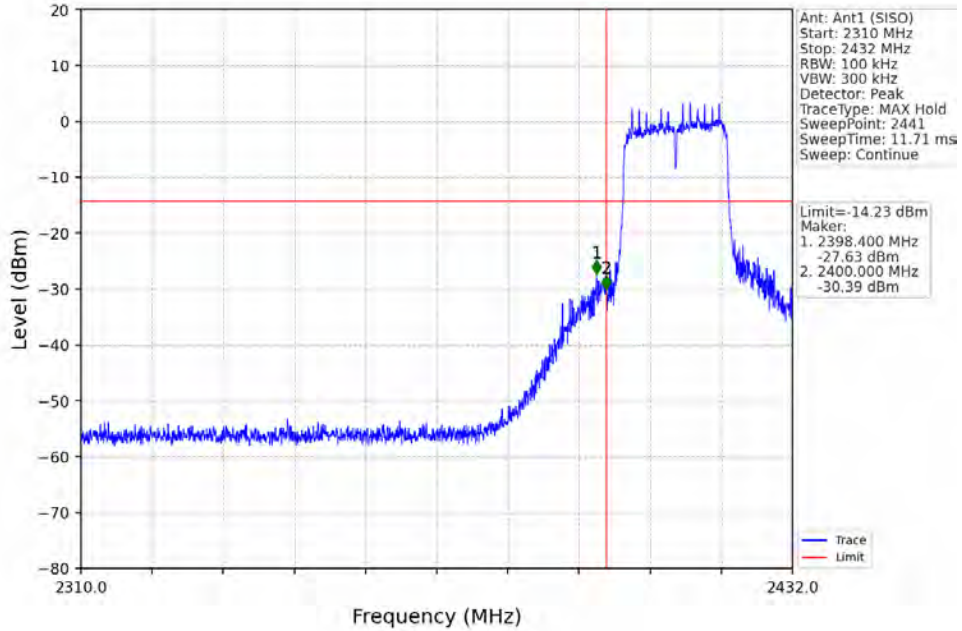
802.11n(HT20)_LCH_2412MHz_Ant1 (SISO)_NTNV
