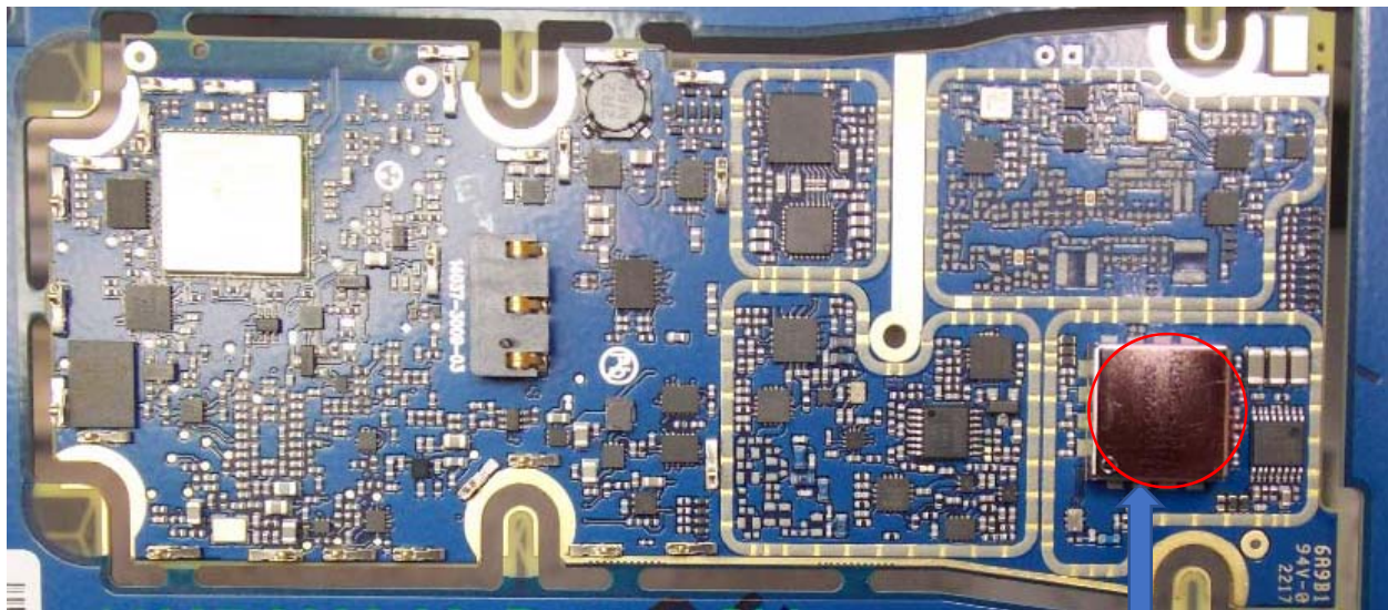
BT/WiFi Module
