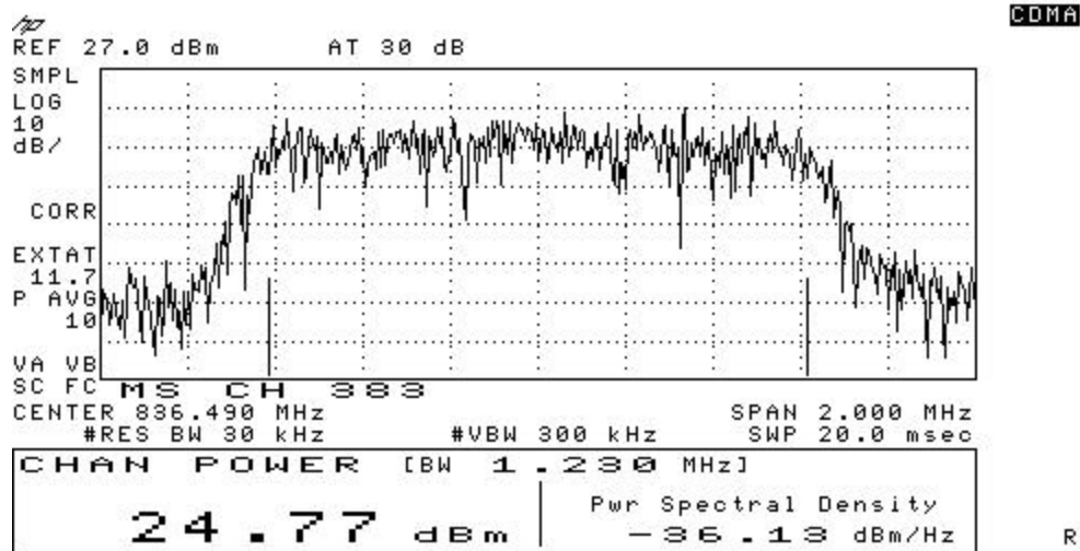
CDMA-800
