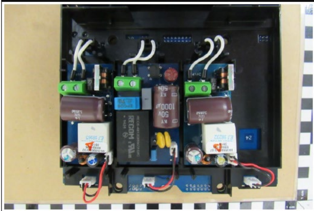
MULTICAL® 803 PCB
