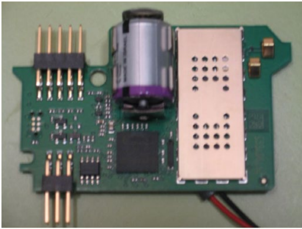
55501605revF1_Front
