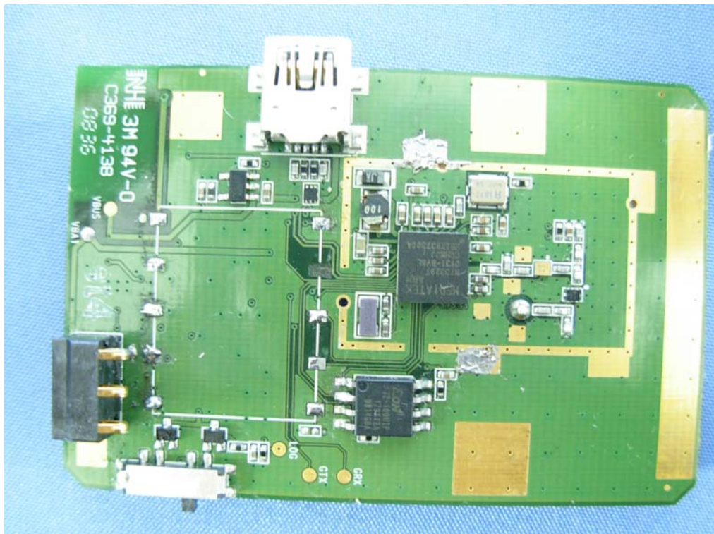
(18) EUT Photo
