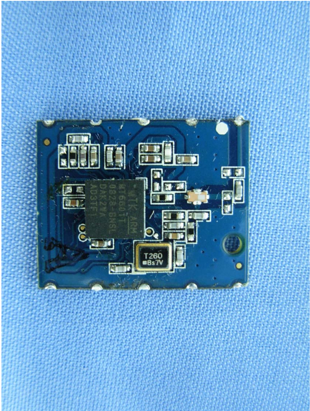
(21) EUT Photo
