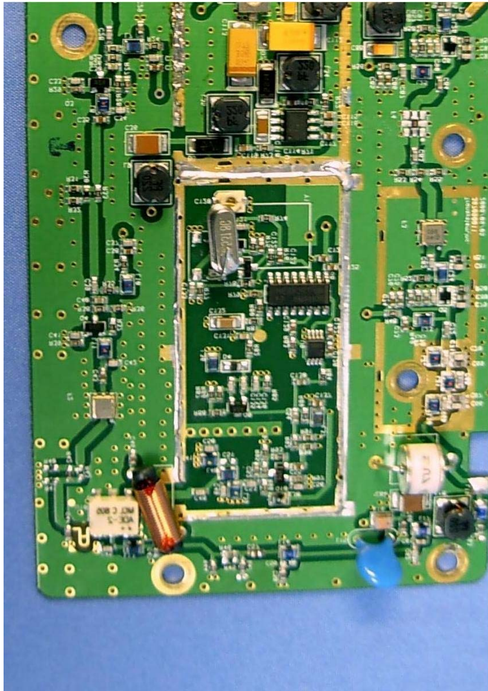
(13) EUT Photo
