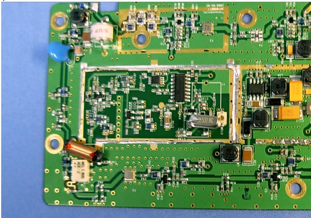
(12) EUT Photo
