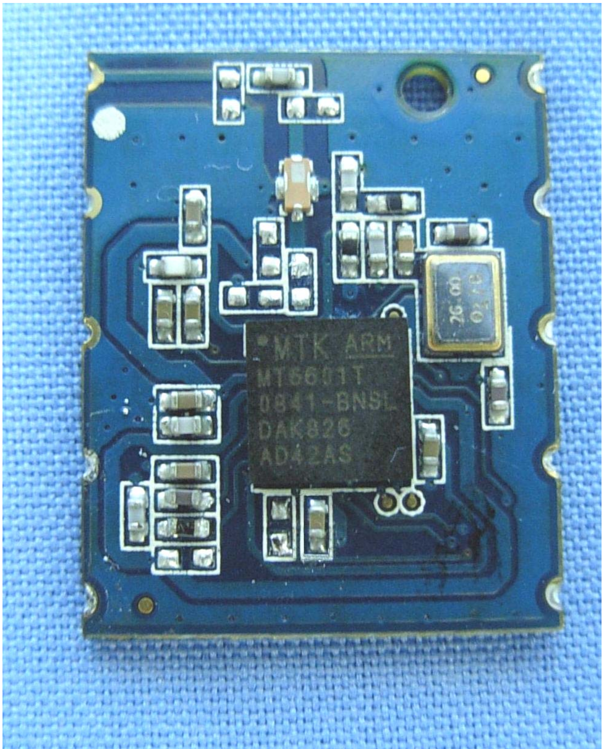
(14) EUT Photo
