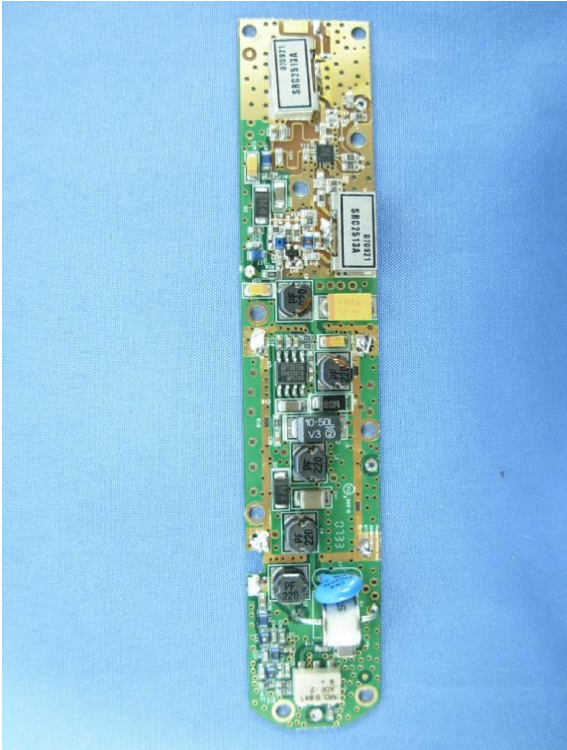
(14) EUT Photo
