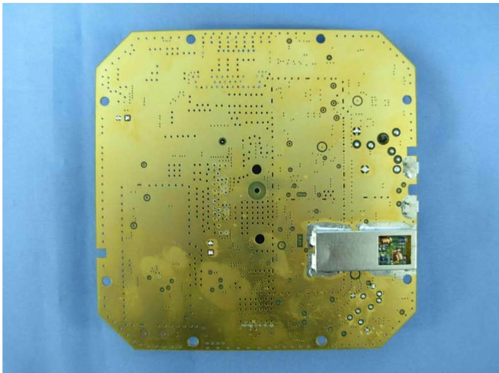
(10) EUT Photo
