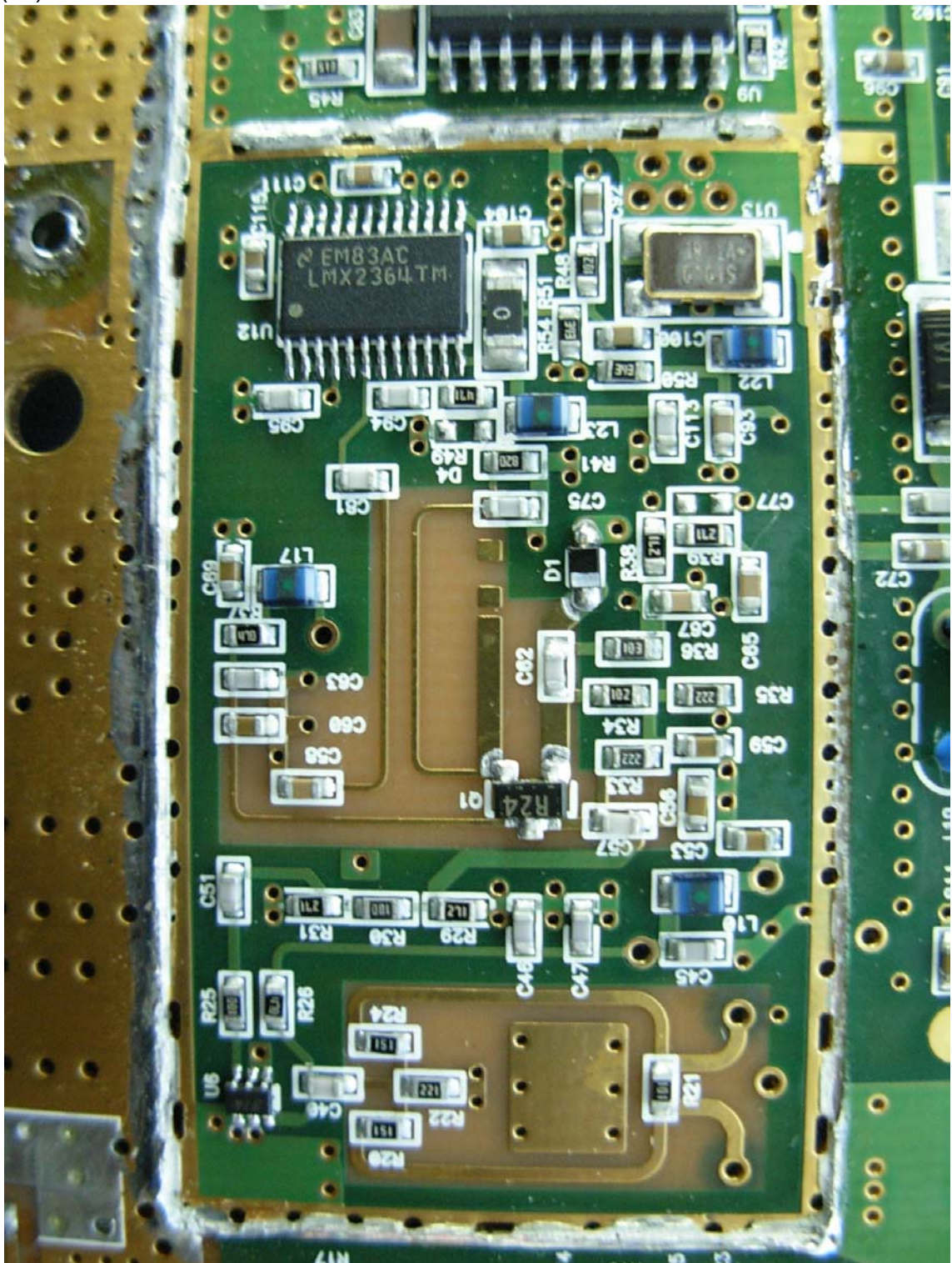
(16) EUT Photo
