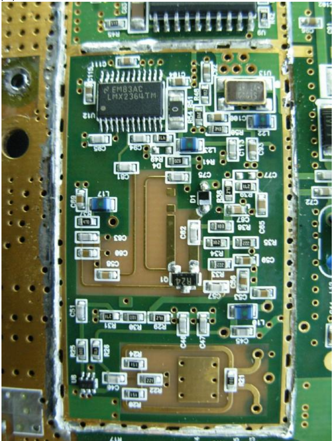
(16) EUT Photo
