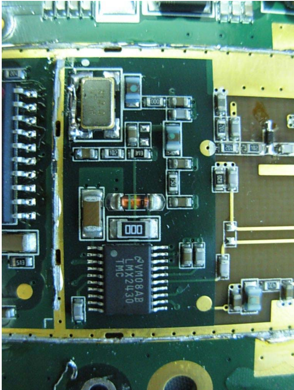
(11) EUT Photo-MB
