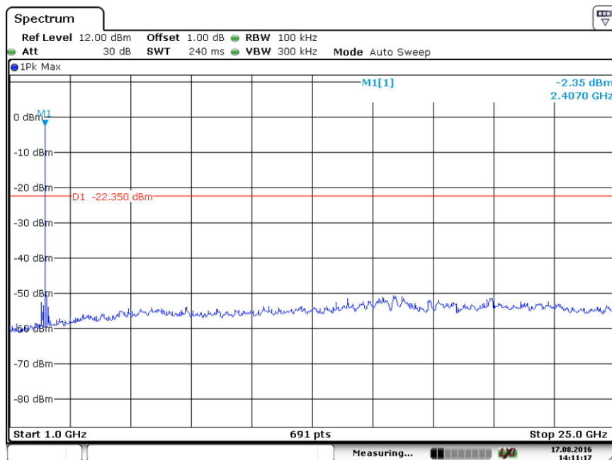
1GHz – 25GHz
