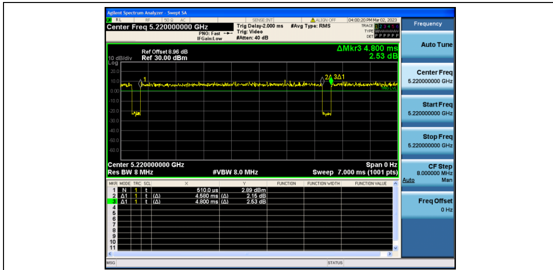
11N20SISO_Ant2_5220
