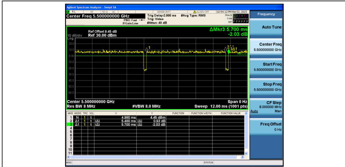
11A_Ant2_5500
