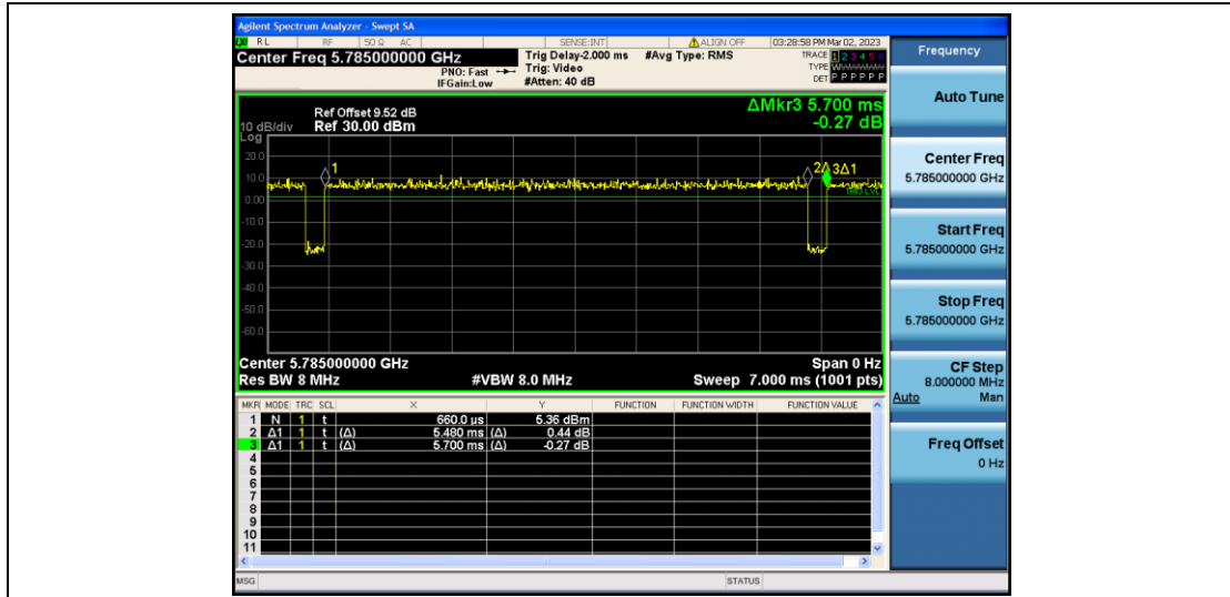
11A_Ant2_5785
