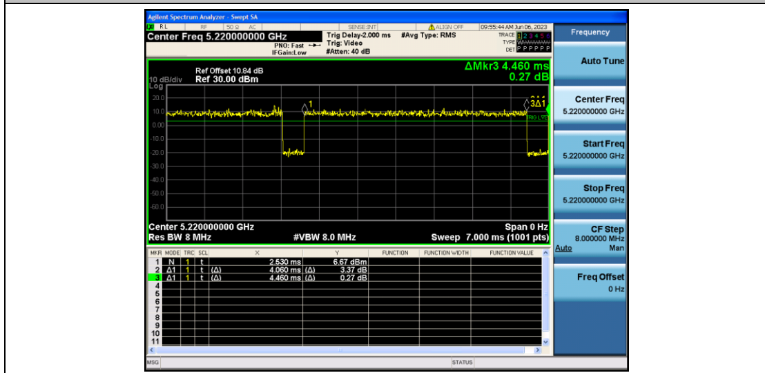
11A_Ant1_5240
