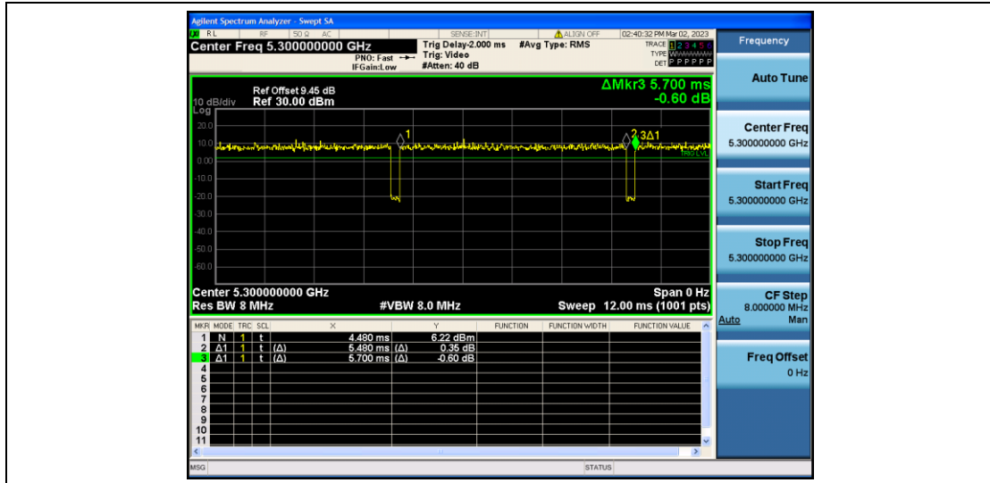
11A_Ant2_5300
