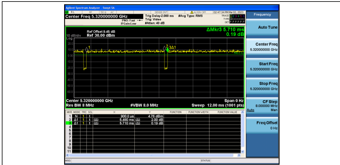
11A_Ant2_5320
