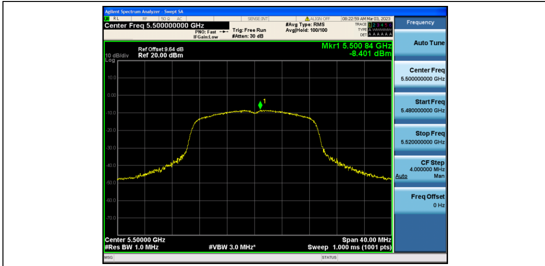
11N20SISO_Ant2_5500
