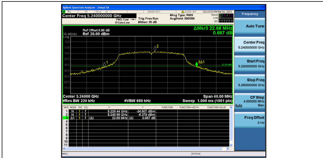
11A_Ant2_5240
