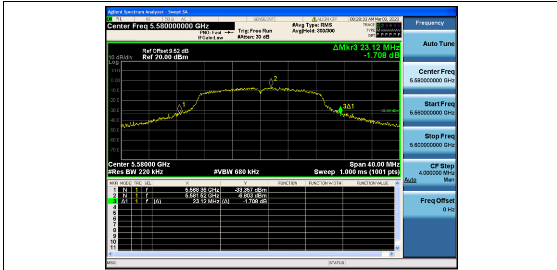
11N20SISO_Ant2_5580
