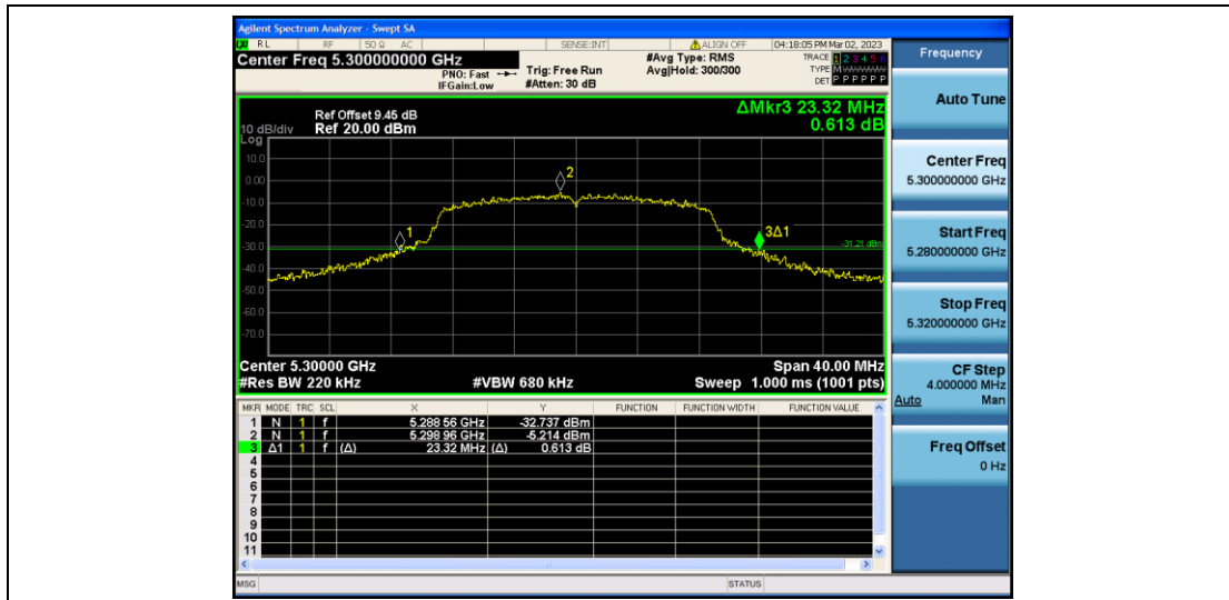
11N20SISO_Ant2_5300
