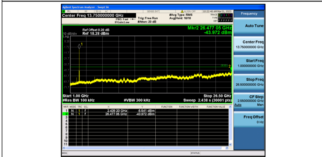
11N20MIMO_Ant2_2437_0~Reference
