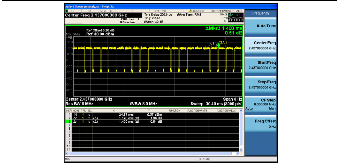
11N20MIMO_Ant2_2437
