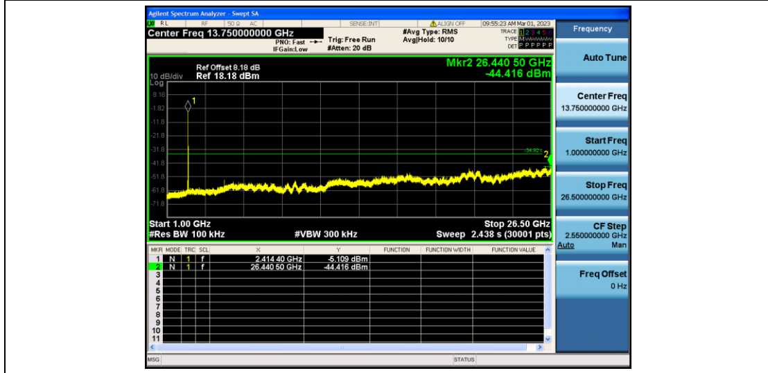
11N20MIMO_Ant2_2412_0~Reference
