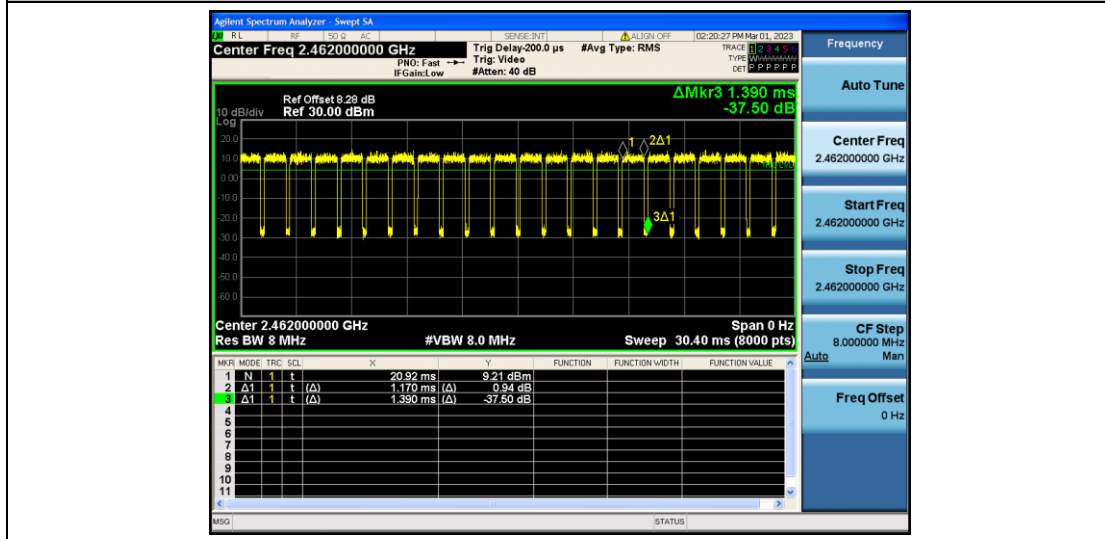
11N20MIMO_Ant2_2462
