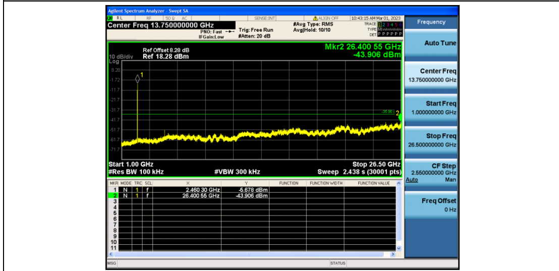
11N20MIMO_Ant2_2462_0~Reference
