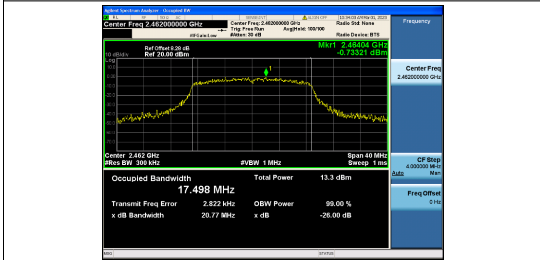
11N20MIMO_Ant2_2462
