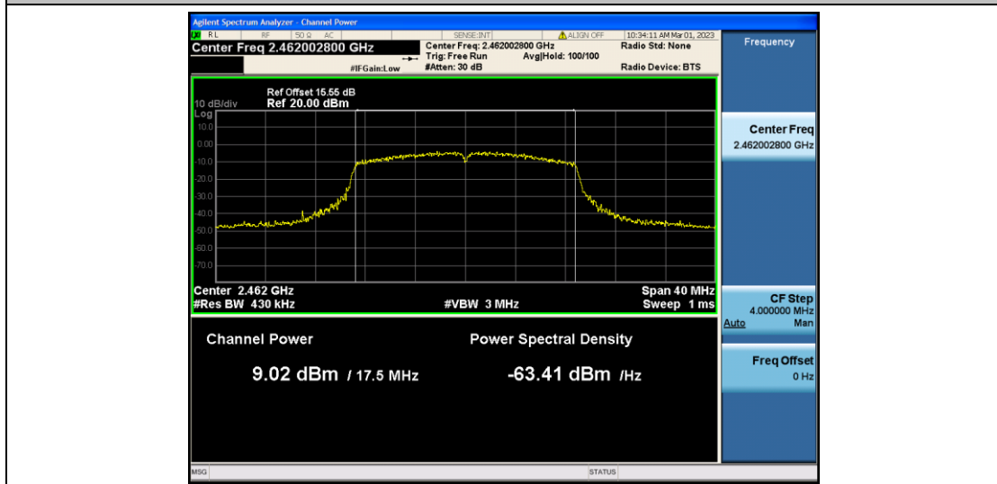
11N20MIMO_Ant2_2462
