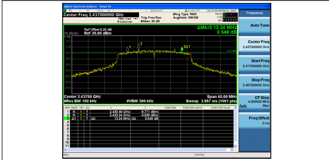
11N20MIMO_Ant2_2437
