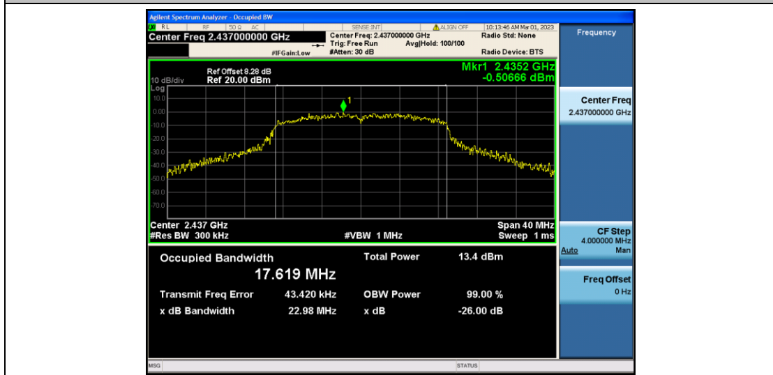
11N20MIMO_Ant2_2437
