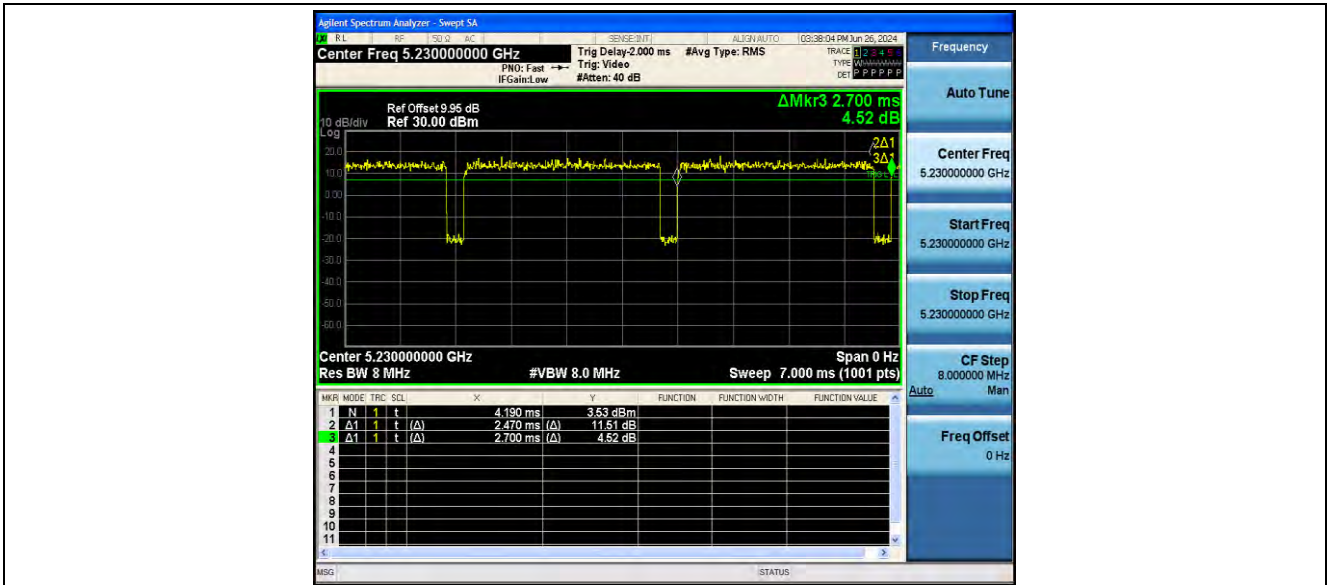
11N40SISO_Ant2_5230
