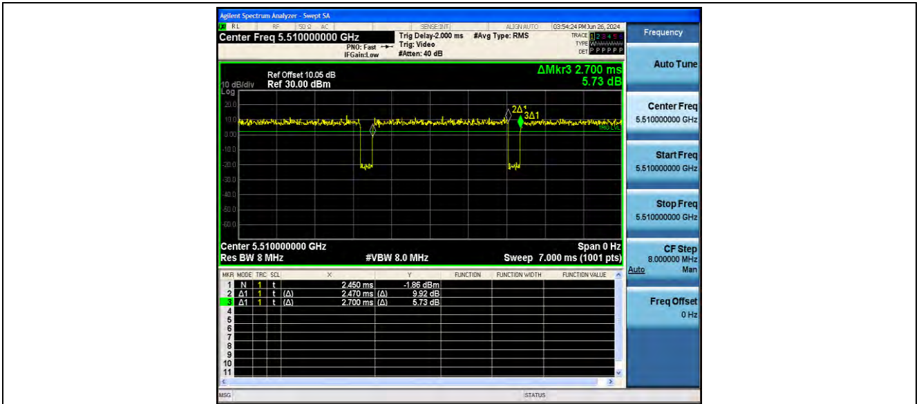
11N40SISO_Ant2_5510
