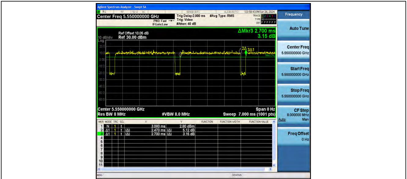
11N40SISO_Ant2_5550
