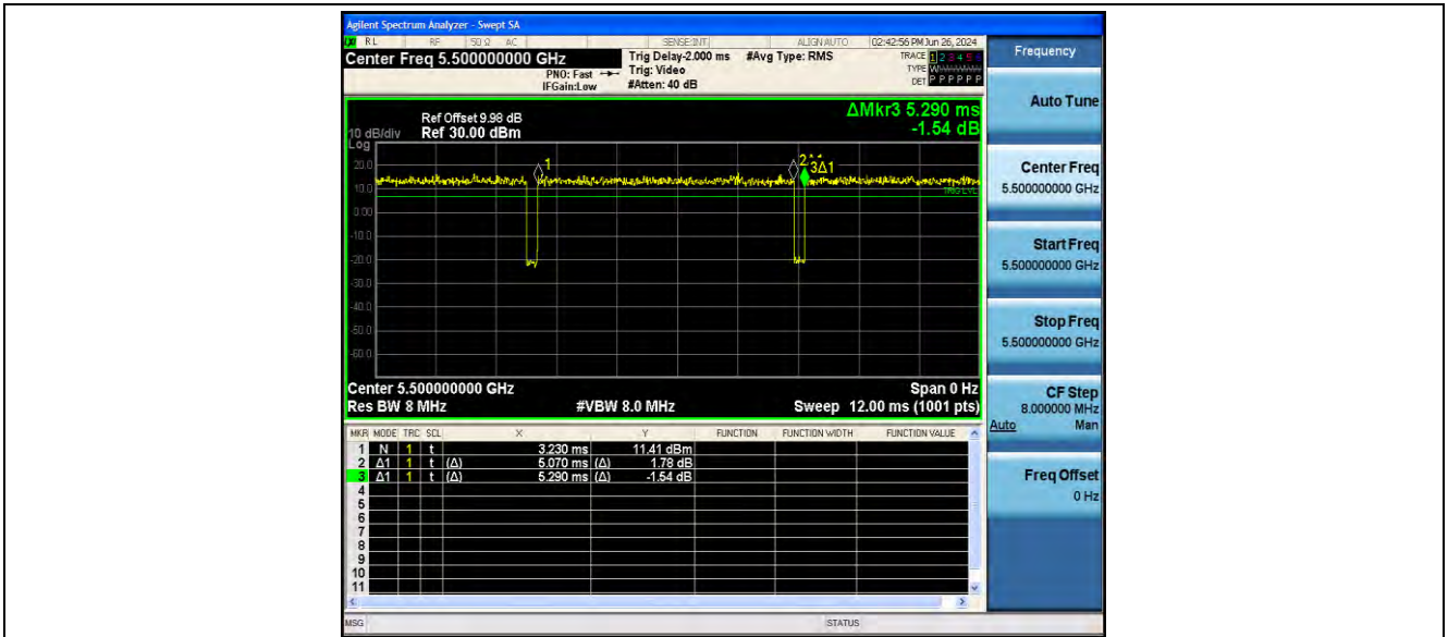
11N20SISO_Ant2_5500
