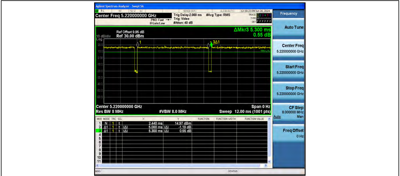
11N20SISO_Ant2_5220
