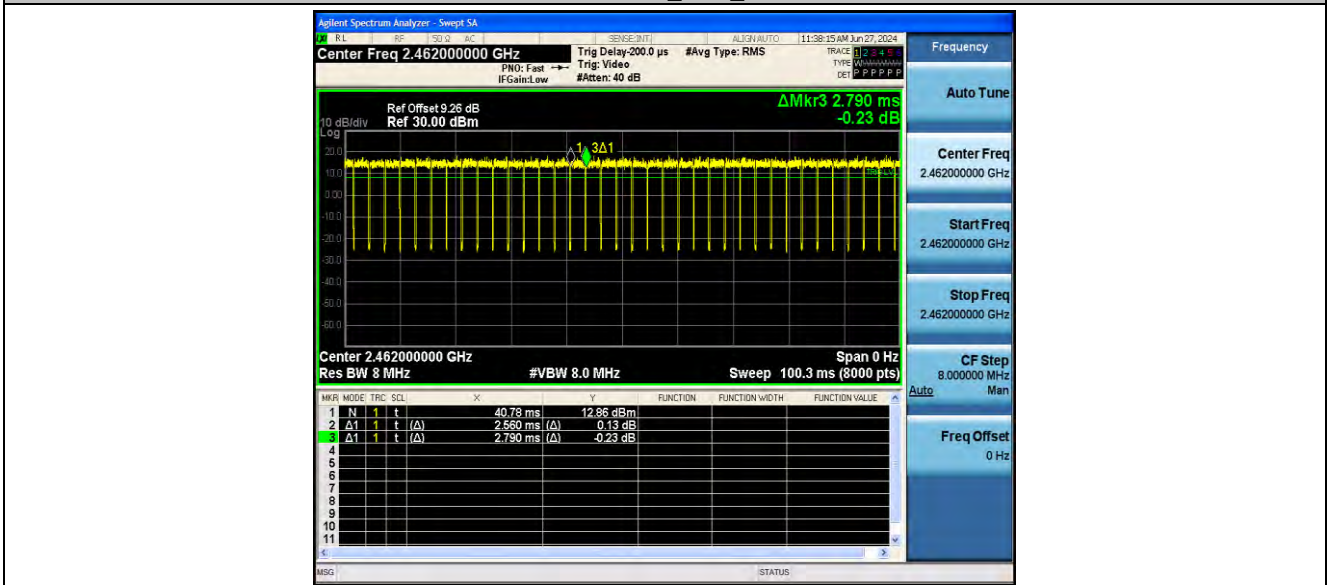
11N20MIMO_Ant1_2462
