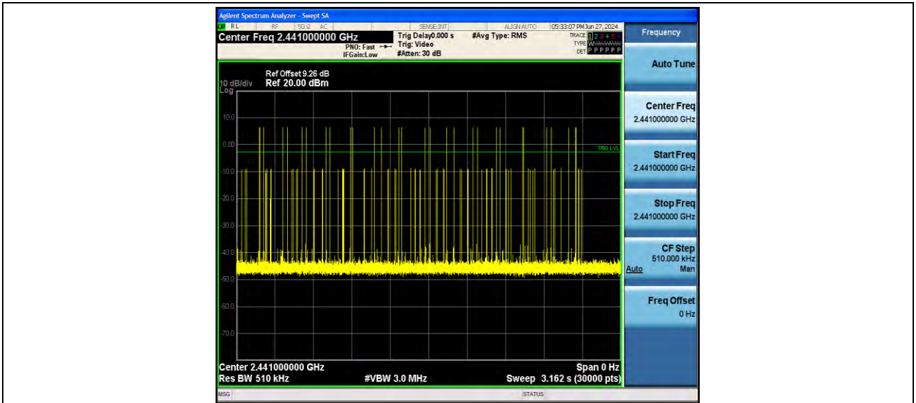
3DH3_Ant1_Hop
