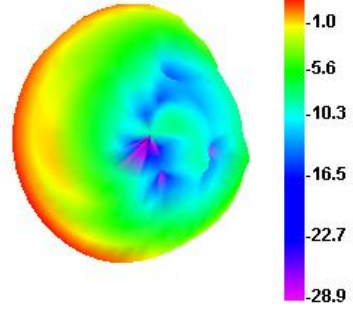
2500.000MHz
