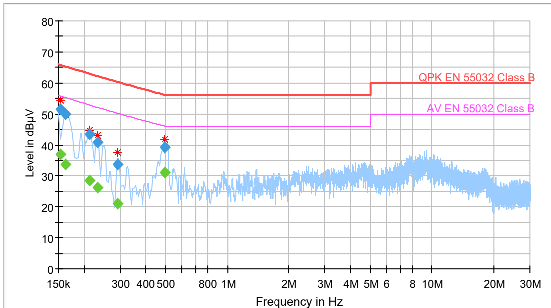
— Preview Result 1-PK+ * Critical_Freqs PK+ — QPK EN 55032 Class B — AV EN 55032 Class B ◆ Final_Result QPK ◆ Final_Result AVG
