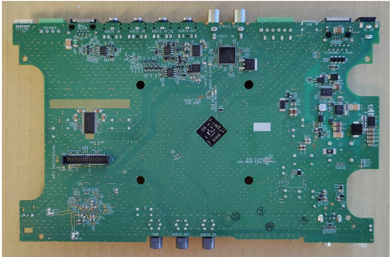
PCB Bottom
