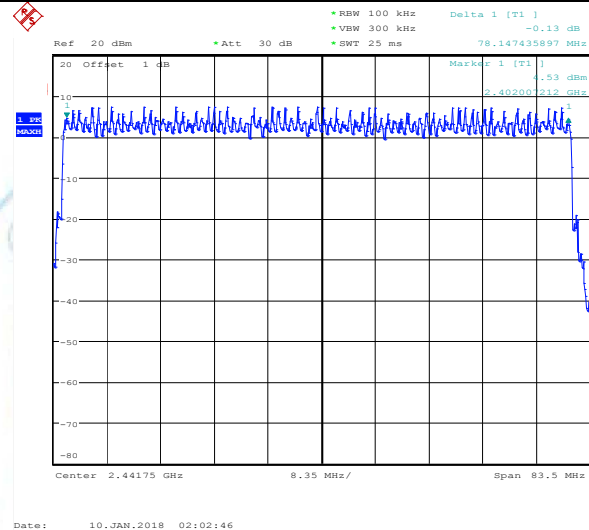
\pi/4 DQPSK Modulation
