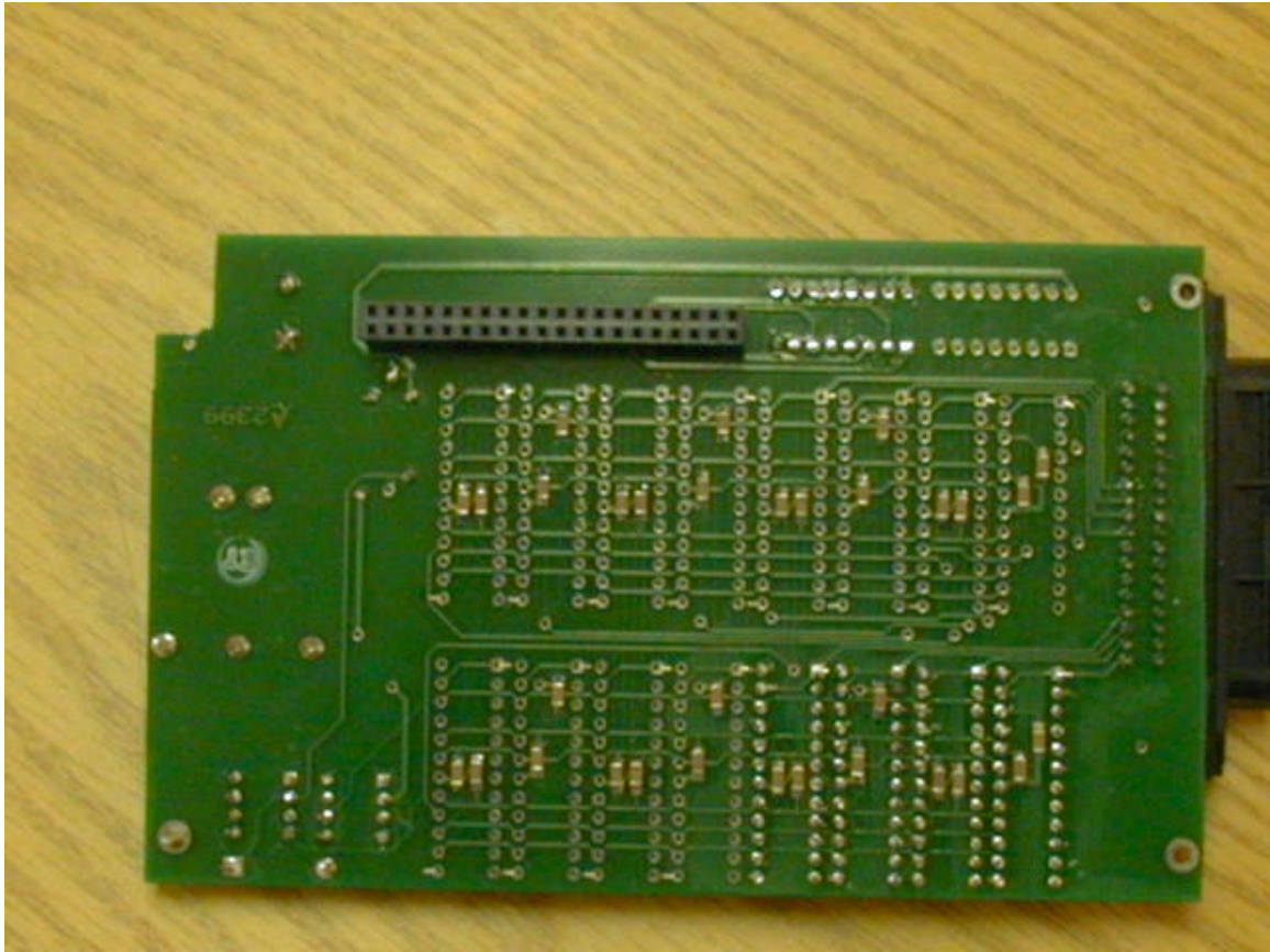
AO-301 Bottom Side
