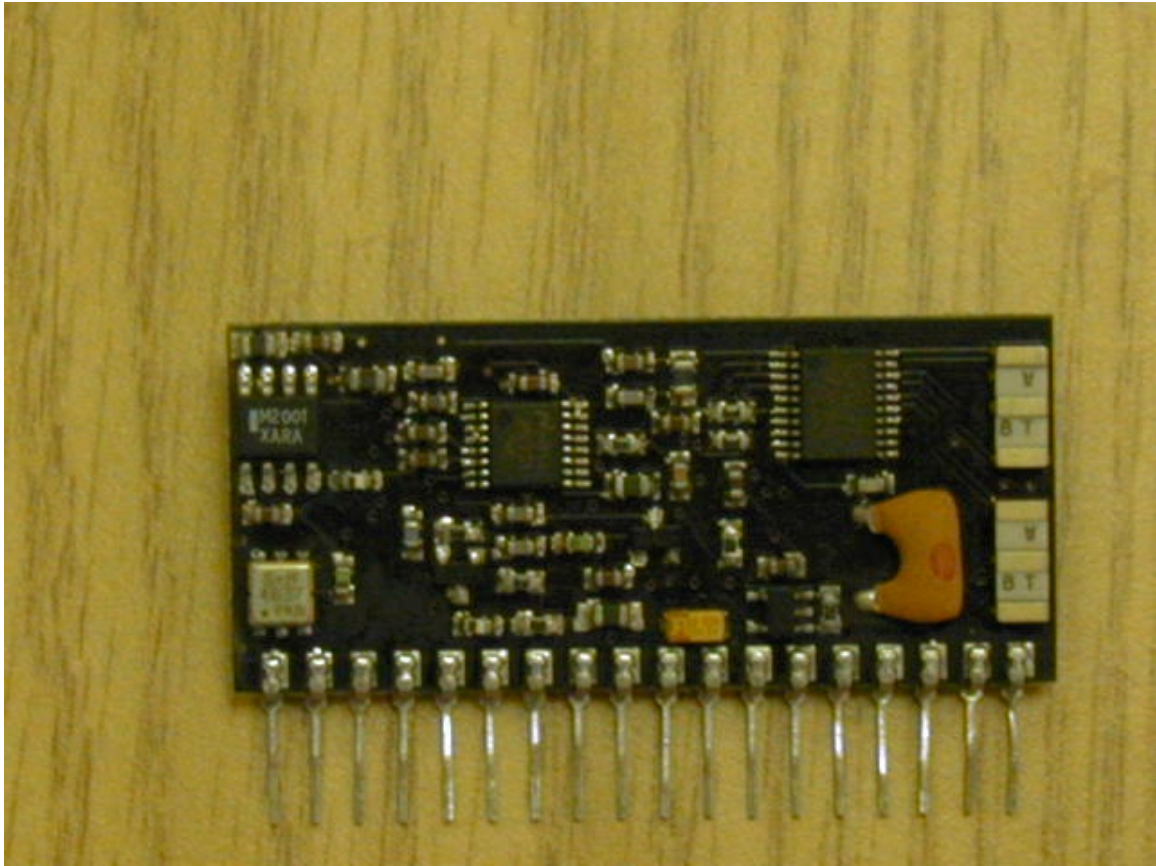
Linx HP-RXM II Bottom Side
