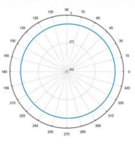
Total-Polar-H-920MHZ
