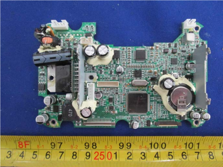
EUT -PCB Mainboard 01 Top View
