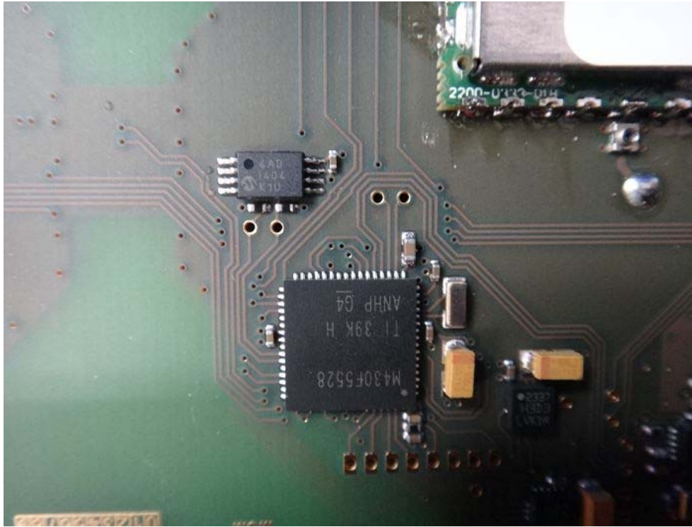
(9) EUT Photo
