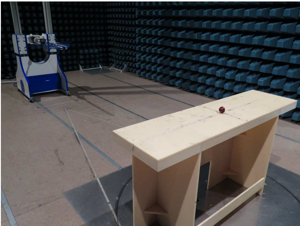
200MHz – 1GHz
