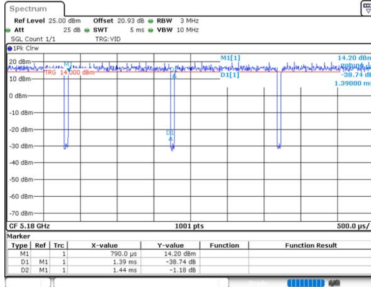
11A_Ant1_5180
