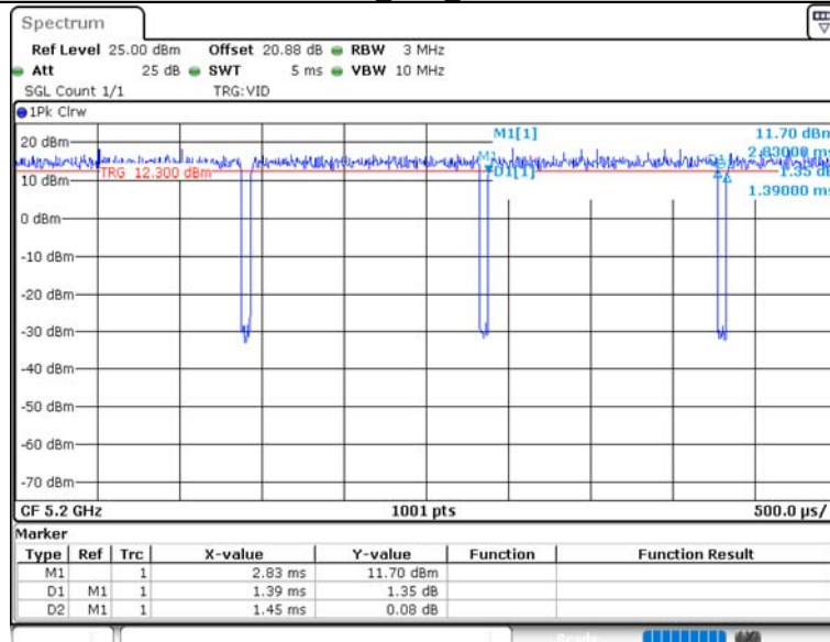
11A_Ant1_5200
