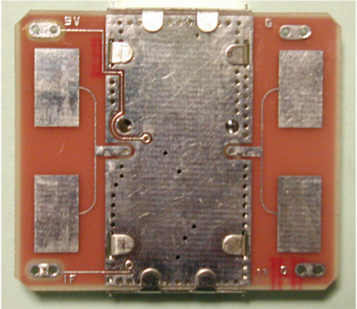
MODULE REAR
