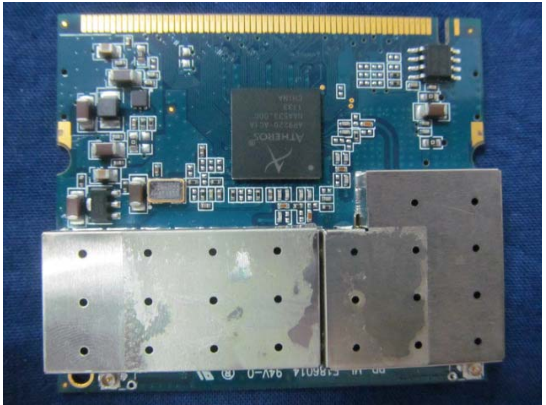
(2) EUT Photo
