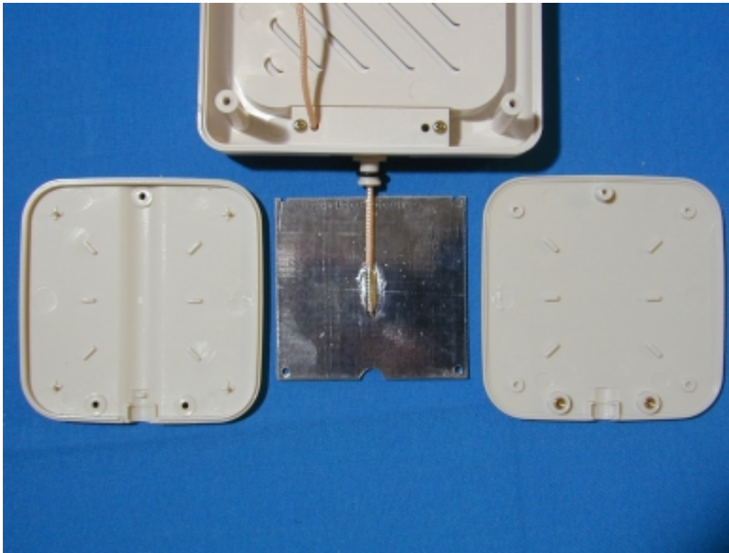
(10) EUT Photo
