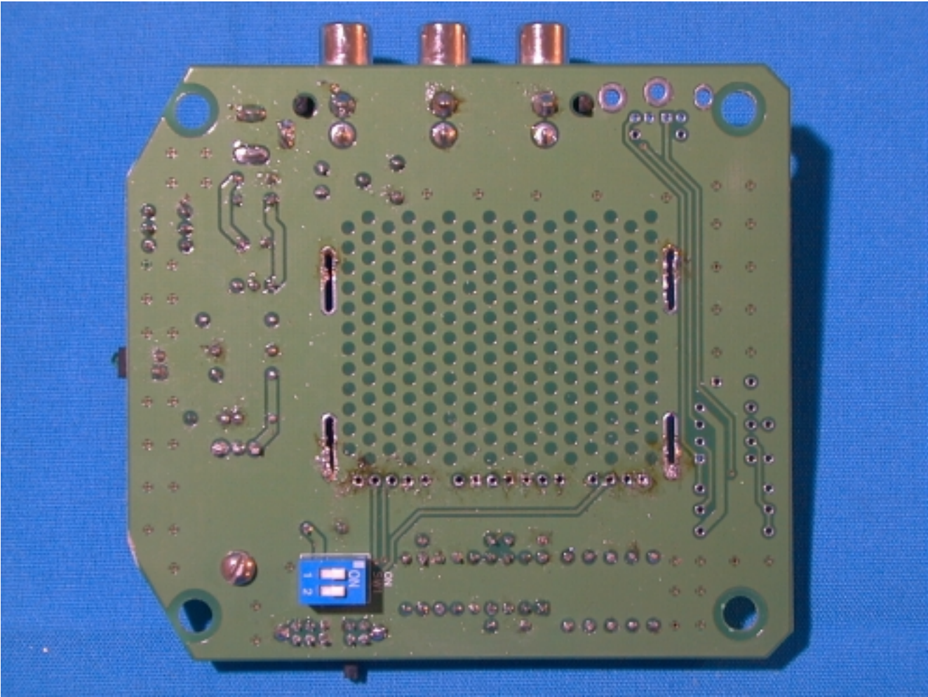
(16) EUT Photo
