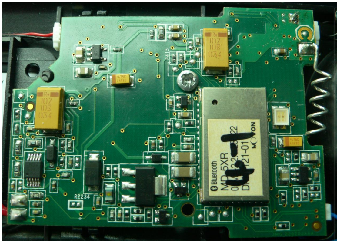
PCB Frontside
