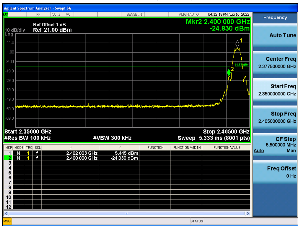
Mode 2 CH00(2402MHz)
