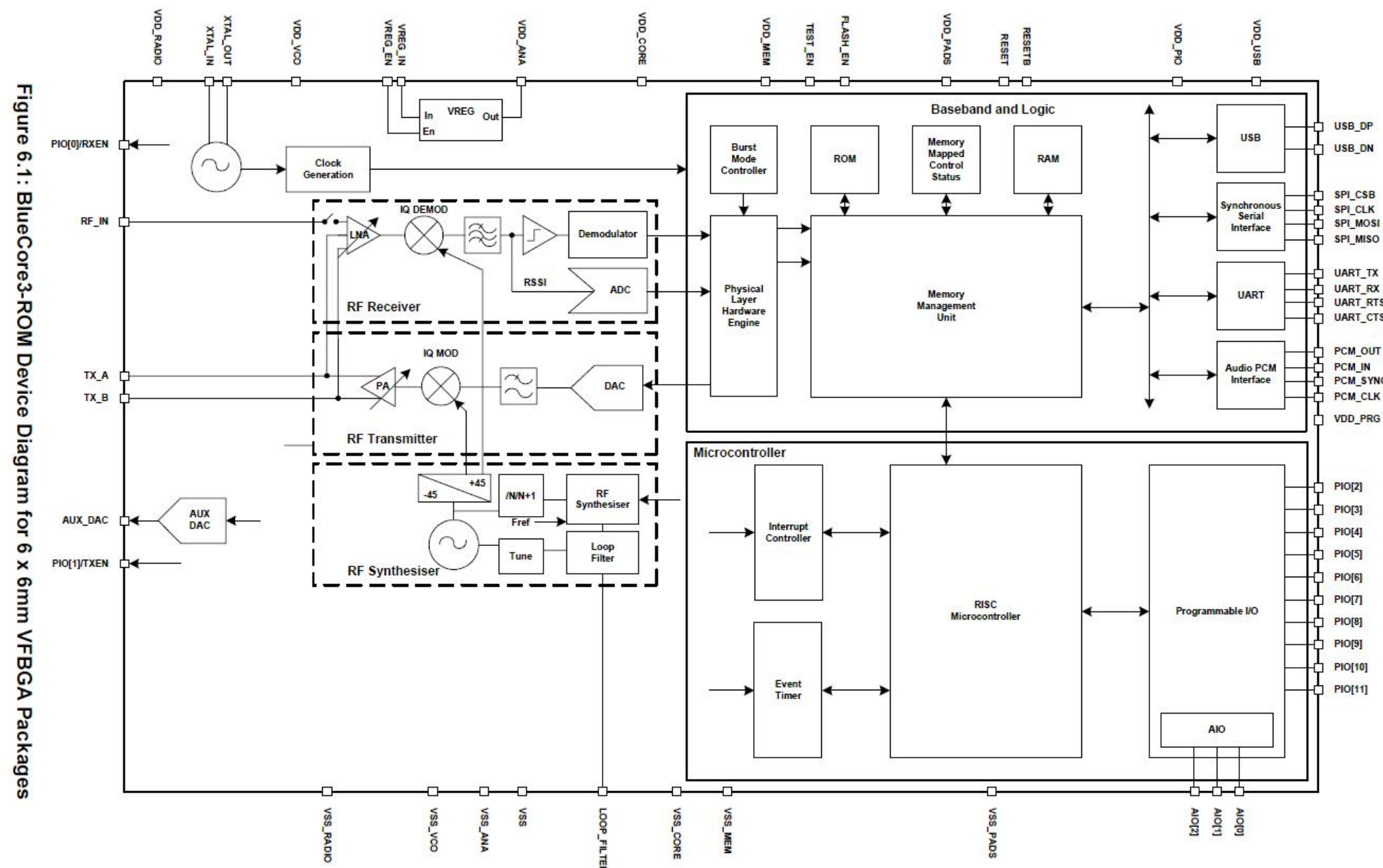
C) BT module block diagram:
