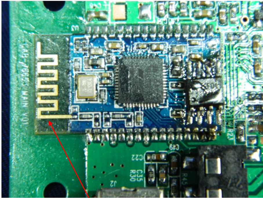
ANTENNA Bluetooth Module
