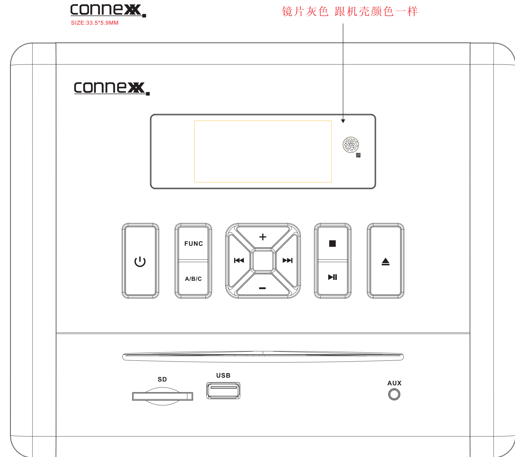
面壳喷油深灰色 面壳丝印：877C
