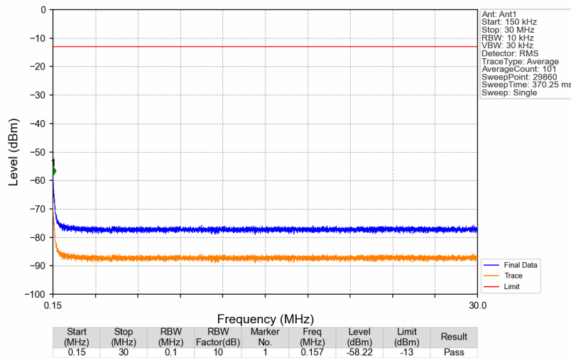
Band26b_881.5MHz_GMSK_SISO_Ant1_NTNV
