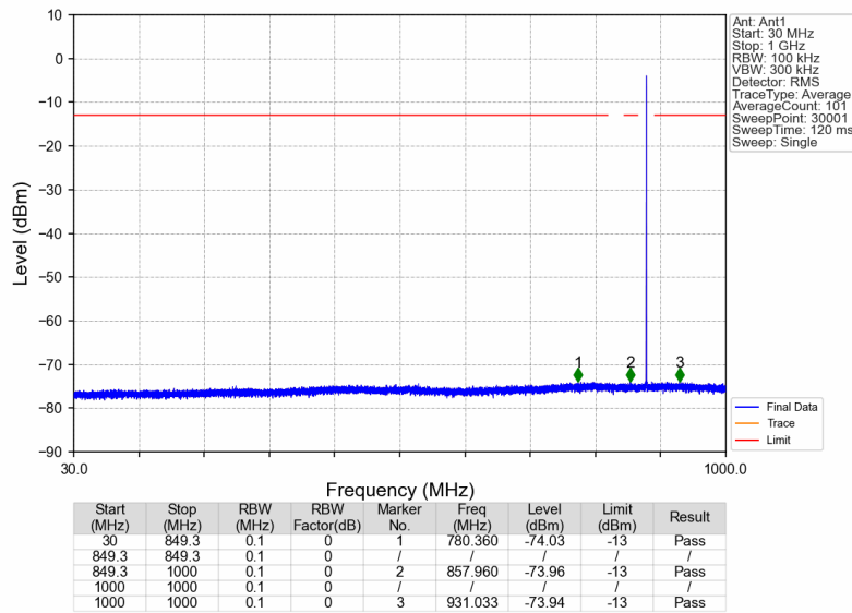
Band26b_881.5MHz_GMSK_SISO_Ant1_NTNV
