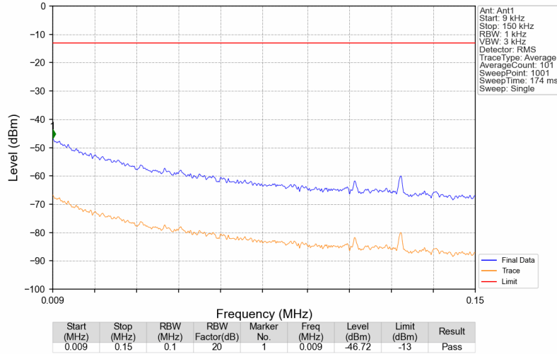
Band26b_891.5MHz_AWGN_SISO_Ant1_NTNV
