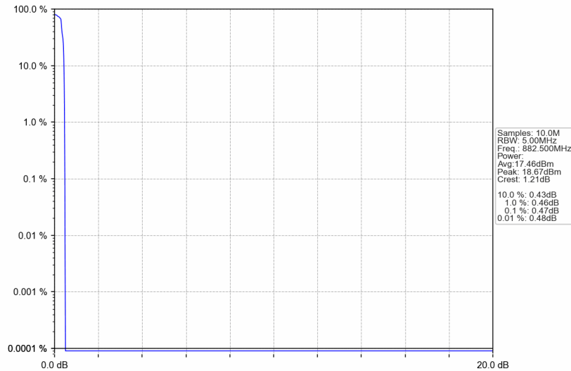
Band26b_882.5MHz_GMSK_SISO_Ant1_NTNV_AGC
