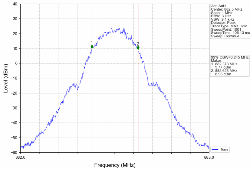
Band26b_882.5MHz_GMSK_SISO_Ant1_NTNV_AGC
