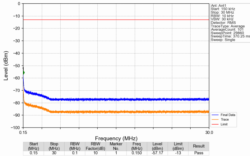
Band26b_881.5MHz_AWGN_SISO_Ant1_NTNV
