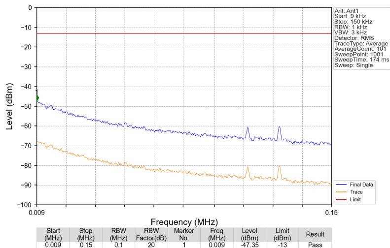
Band26b_893.9MHz_GMSK_SISO_Ant1_NTNV
