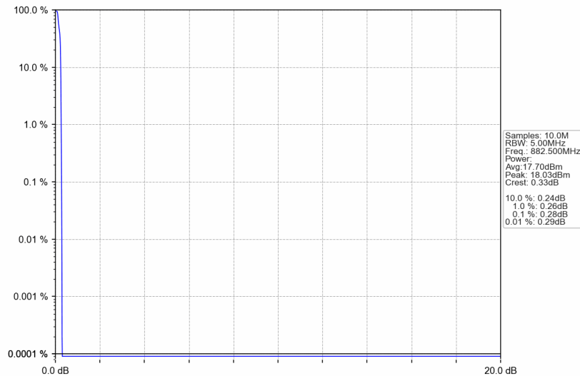
Band26b_882.5MHz_GMSK_SISO_Ant1_NTNV_AGC+3
