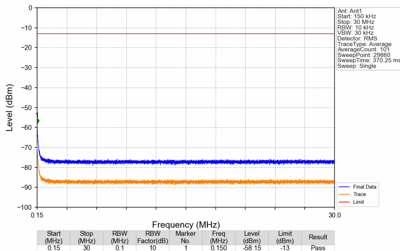
Band26b_893.9MHz_GMSK_SISO_Ant1_NTNV
