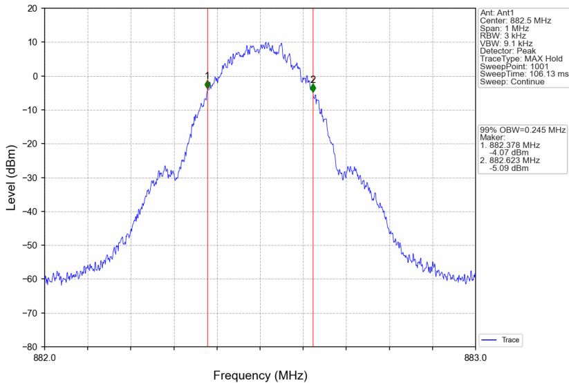
Band26b_882.5MHz_GMSK_SISO_Ant1_NTNV_AGC+3
