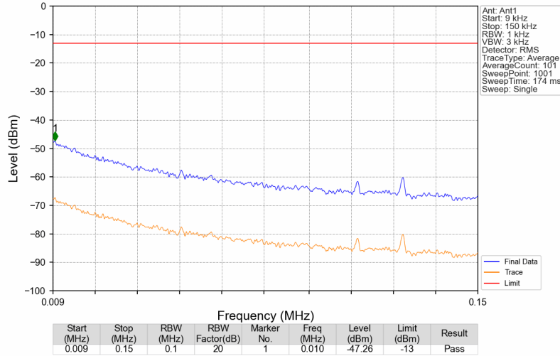
Band26b_881.5MHz_AWGN_SISO_Ant1_NTNV
