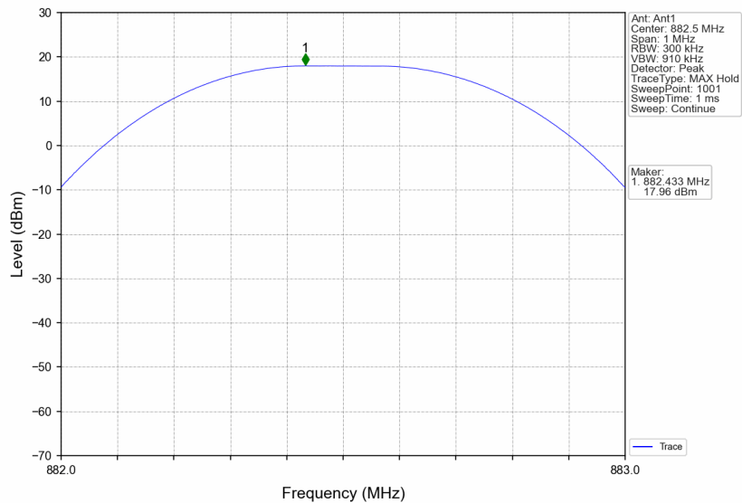
Band26b_882.5MHz_GMSK_SISO_Ant1_NTNV_AGC+3
