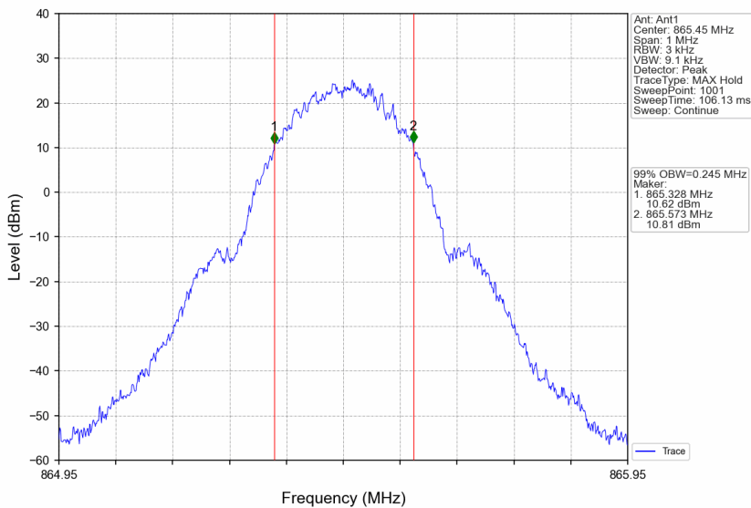
Band26a_865.45MHz_GMSK_SISO_Ant1_NTNV_AGC
