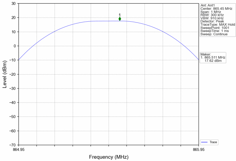
Band26a_865.45MHz_GMSK_SISO_Ant1_NTNV_AGC+3
