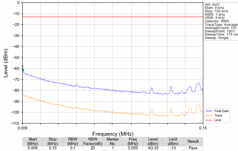
Band26a_868.9MHz_GMSK_SISO_Ant1_NTNV
