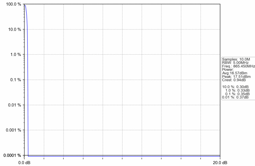
Band26a_865.45MHz_GMSK_SISO_Ant1_NTNV_AGC
