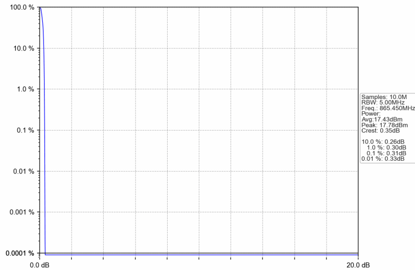
Band26a_865.45MHz_GMSK_SISO_Ant1_NTNV_AGC+3
