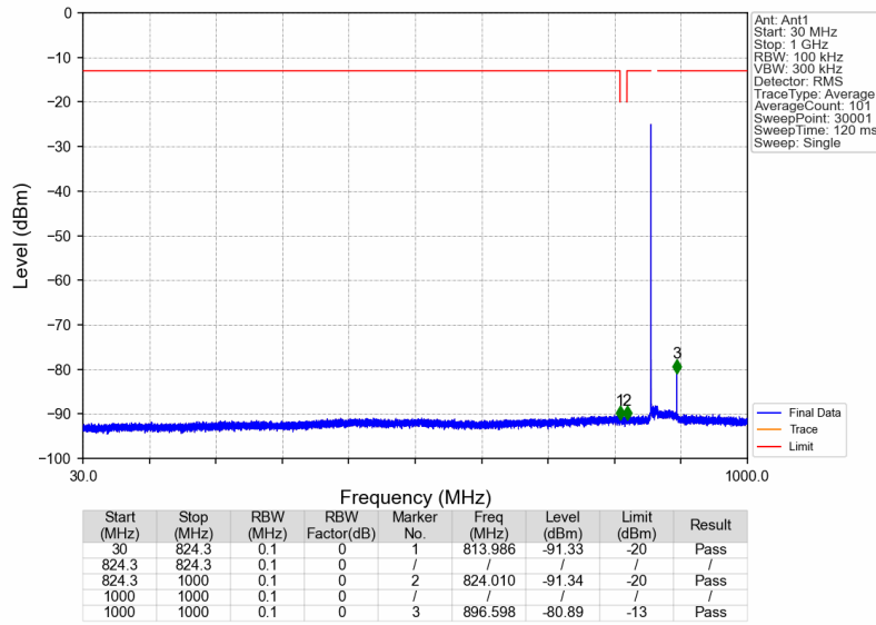
Band26a_859.1MHz_GMSK_SISO_Ant1_NTNV
