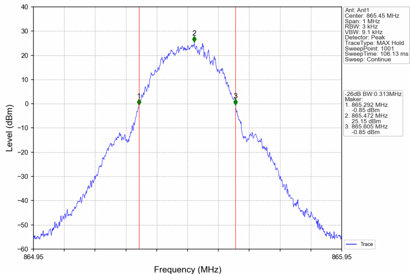
Band26a_865.45MHz_GMSK_SISO_Ant1_NTNV_AGC
