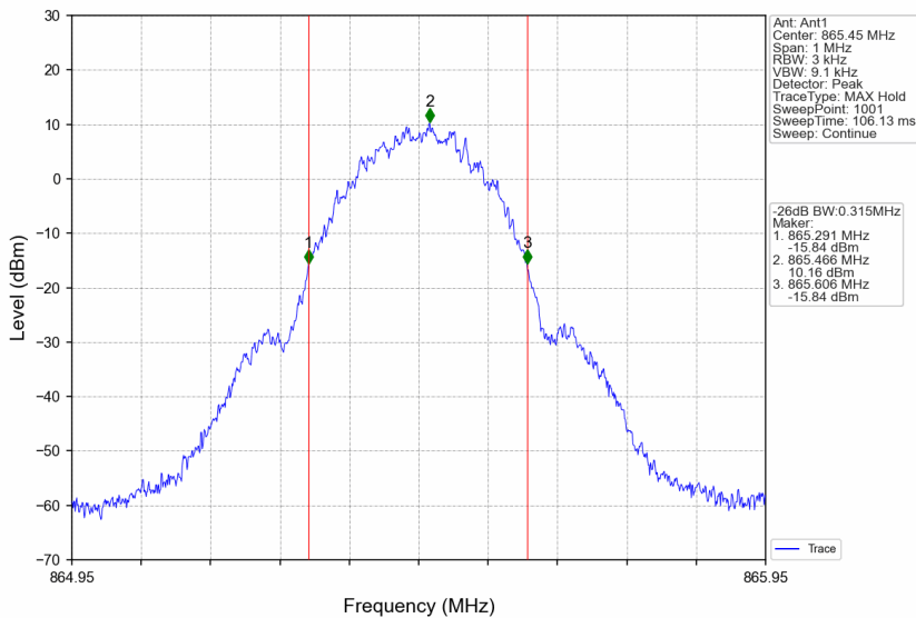
Band26a_865.45MHz_GMSK_SISO_Ant1_NTNV_AGC+3
