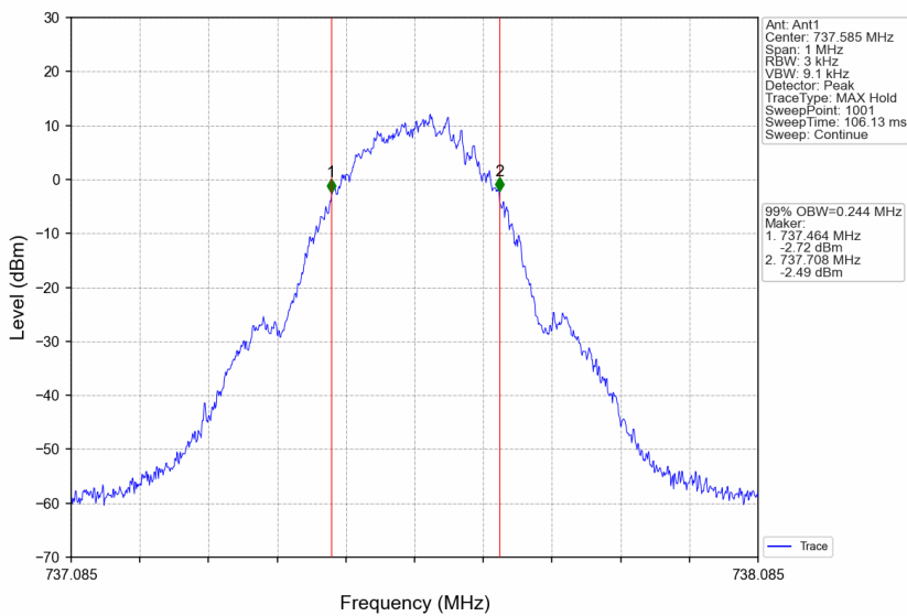
Band12_737.585MHz_GMSK_SISO_Ant1_NTNV_AGC+3
