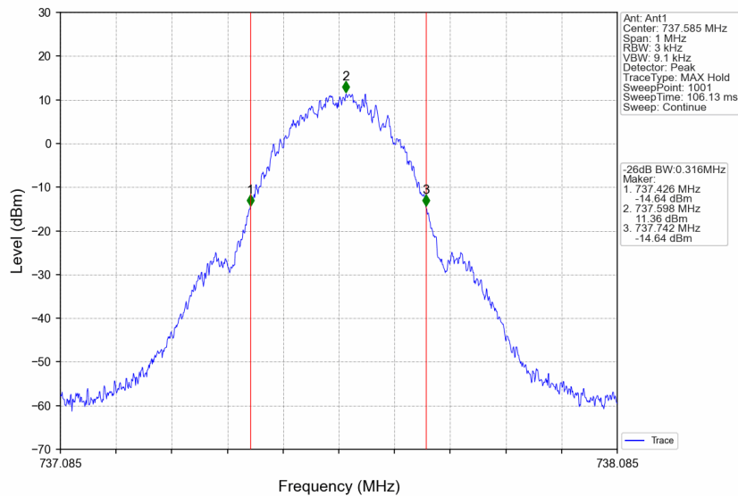
Band12_737.585MHz_GMSK_SISO_Ant1_NTNV_AGC+3
