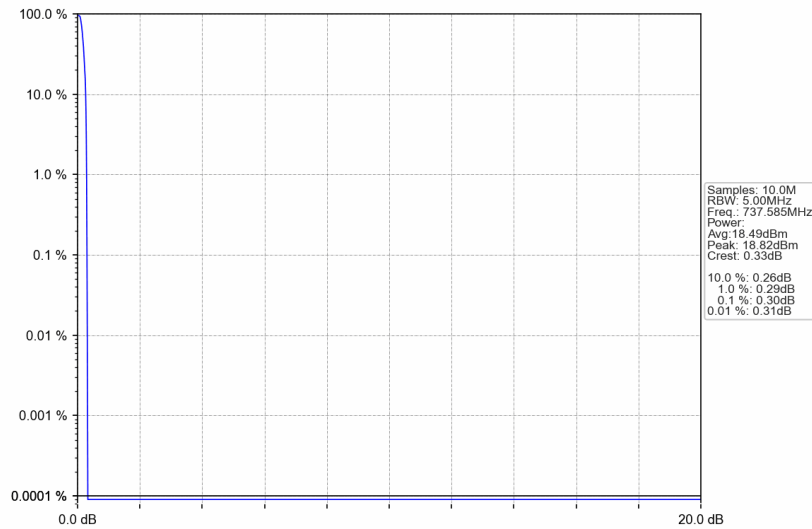
Band12_737.585MHz_GMSK_SISO_Ant1_NTNV_AGC+3
