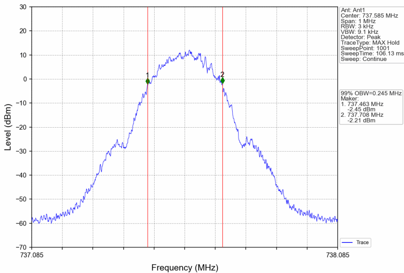
Band12_737.585MHz_GMSK_SISO_Ant1_NTNV_AGC+3
