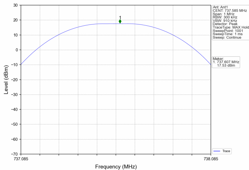
Band12_737.585MHz_GMSK_SISO_Ant1_NTNV_AGC+3
