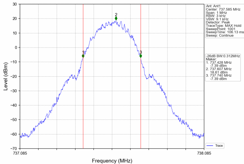
Band12_737.585MHz_GMSK_SISO_Ant1_NTNV_AGC
