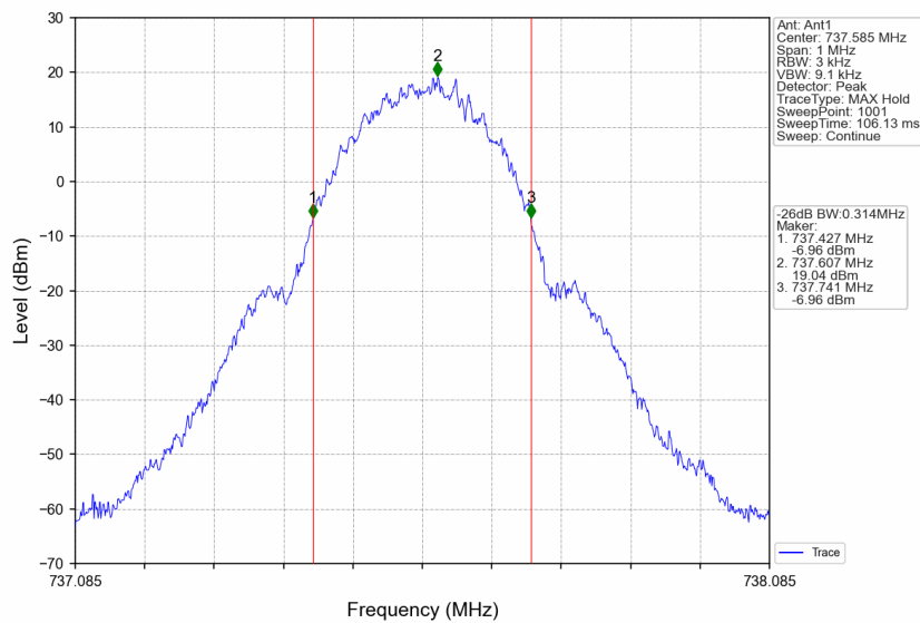
Band12_737.585MHz_GMSK_SISO_Ant1_NTNV_AGC
