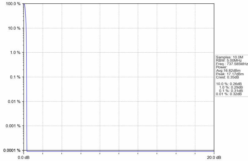
Band12_737.585MHz_GMSK_SISO_Ant1_NTNV_AGC
