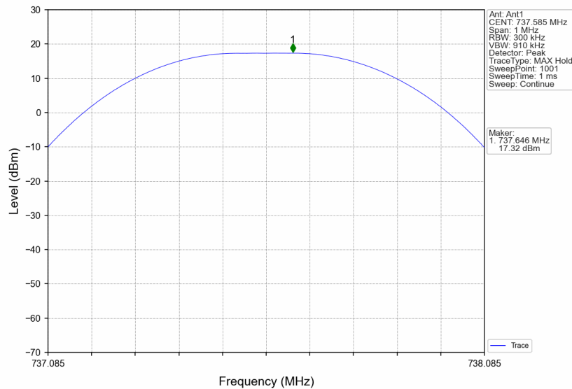
Band12_737.585MHz_GMSK_SISO_Ant1_NTNV_AGC+3
