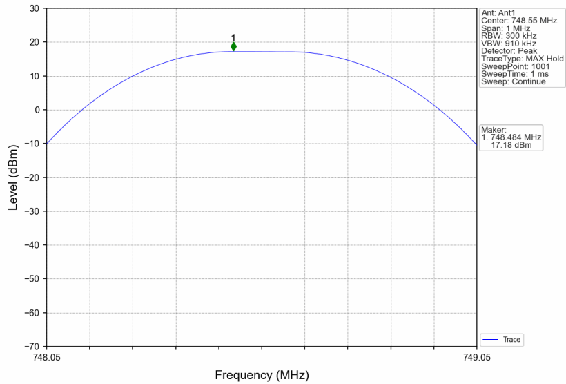
Band13_748.55MHz_GMSK_SISO_Ant1_NTNV_AGC+3
