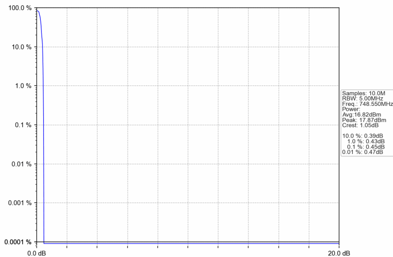
Band13_748.55MHz_GMSK_SISO_Ant1_NTNV_AGC
