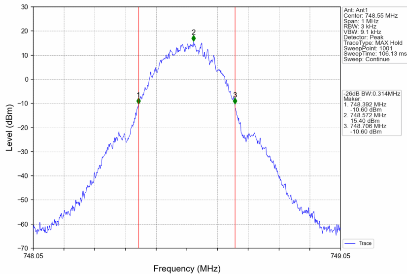
Band13_748.55MHz_GMSK_SISO_Ant1_NTNV_AGC
