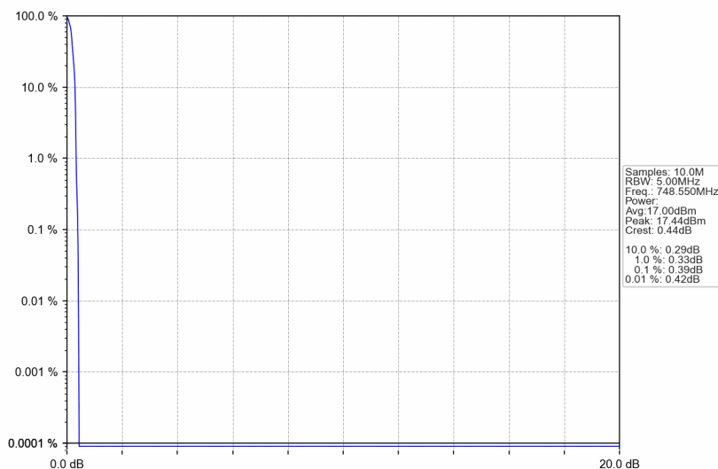
Band13_748.55MHz_GMSK_SISO_Ant1_NTNV_AGC+3
