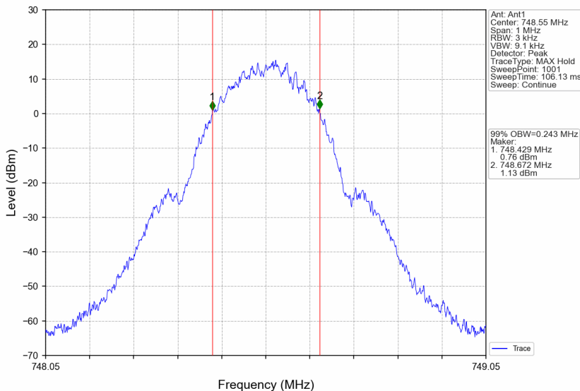
Band13_748.55MHz_GMSK_SISO_Ant1_NTNV_AGC
