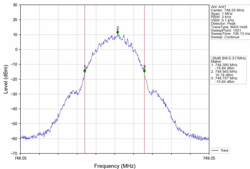
Band13_748.55MHz_GMSK_SISO_Ant1_NTNV_AGC+3
