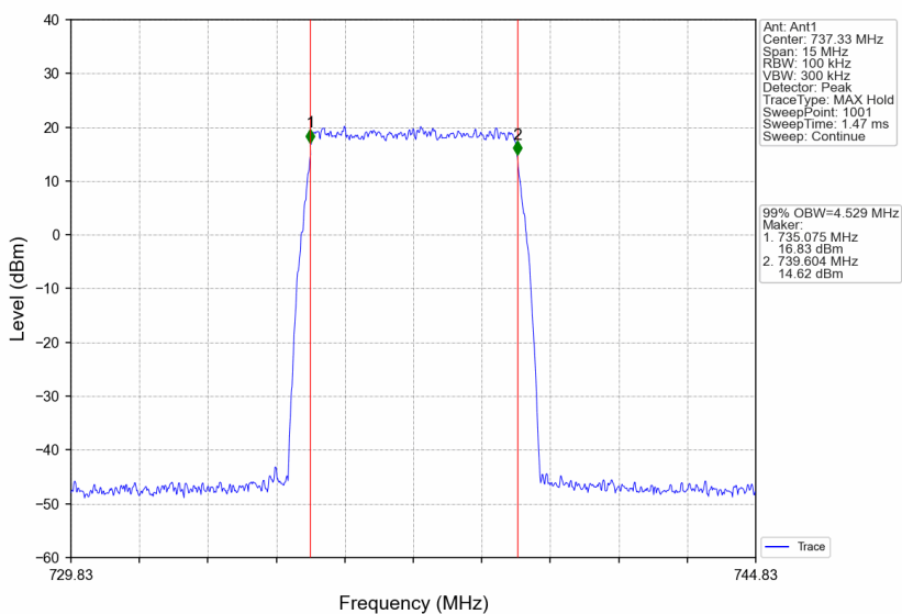
Band12_737.33MHz_AWGN_SISO_Ant1_NTNV_AGC
