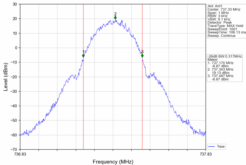
Band12_737.33MHz_GMSK_SISO_Ant1_NTNV_AGC
