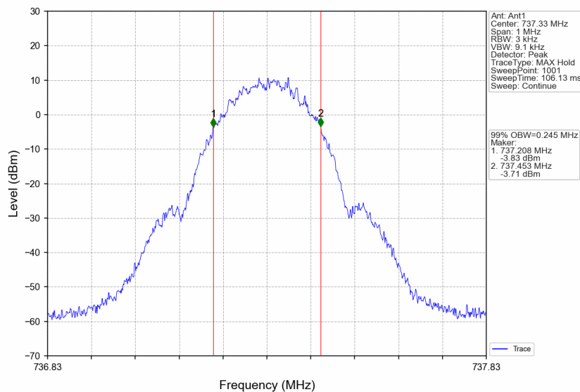
Band12_737.33MHz_GMSK_SISO_Ant1_NTNV_AGC+3
