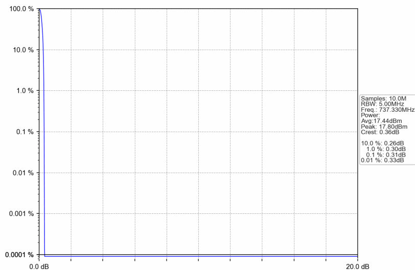
Band12_737.33MHz_GMSK_SISO_Ant1_NTNV_AGC+3
