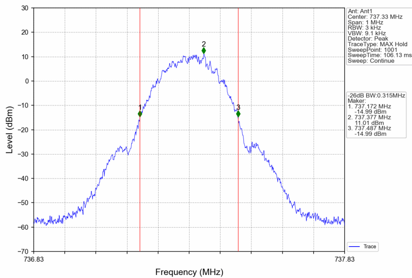
Band12_737.33MHz_GMSK_SISO_Ant1_NTNV_AGC+3
