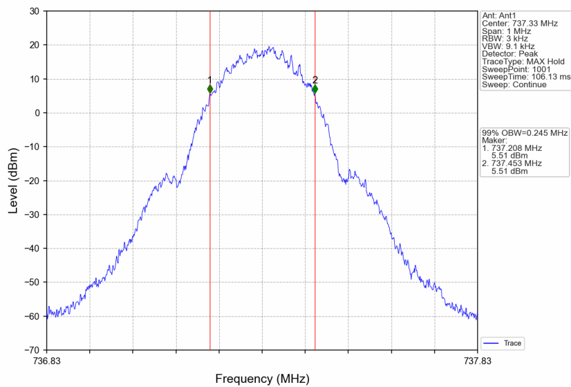
Band12_737.33MHz_GMSK_SISO_Ant1_NTNV_AGC
