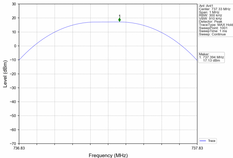
Band12_737.33MHz_GMSK_SISO_Ant1_NTNV_AGC+3
