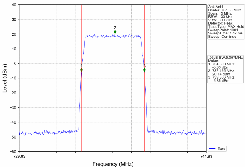
Band12_737.33MHz_AWGN_SISO_Ant1_NTNV_AGC
