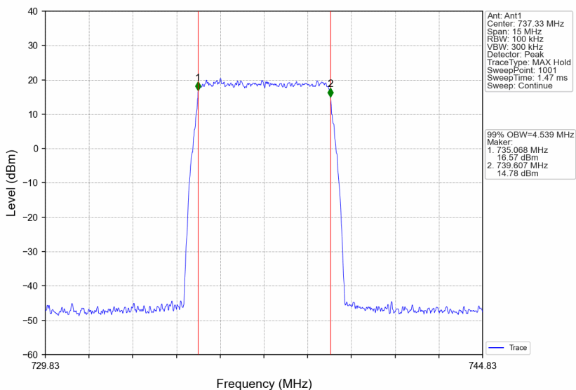
Band12_737.33MHz_AWGN_SISO_Ant1_NTNV_AGC
