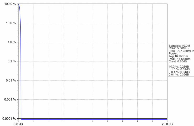
Band12_737.33MHz_GMSK_SISO_Ant1_NTNV_AGC
