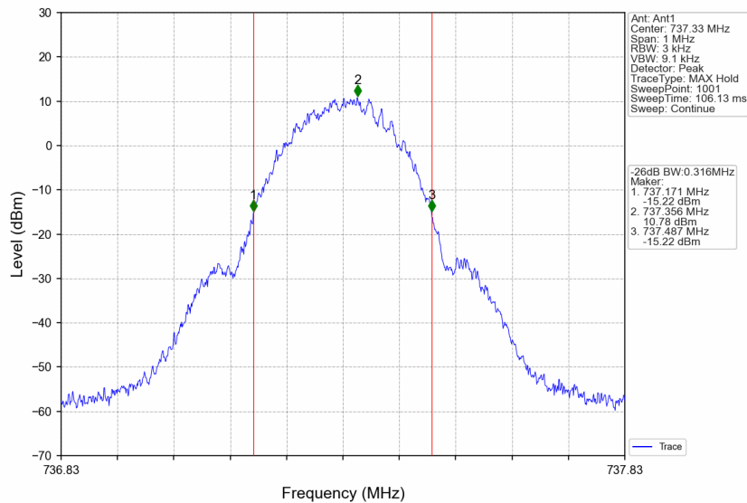
Band12_737.33MHz_GMSK_SISO_Ant1_NTNV_AGC+3
