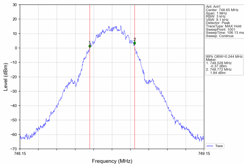
Band13_748.65MHz_GMSK_SISO_Ant1_NTNV_AGC
