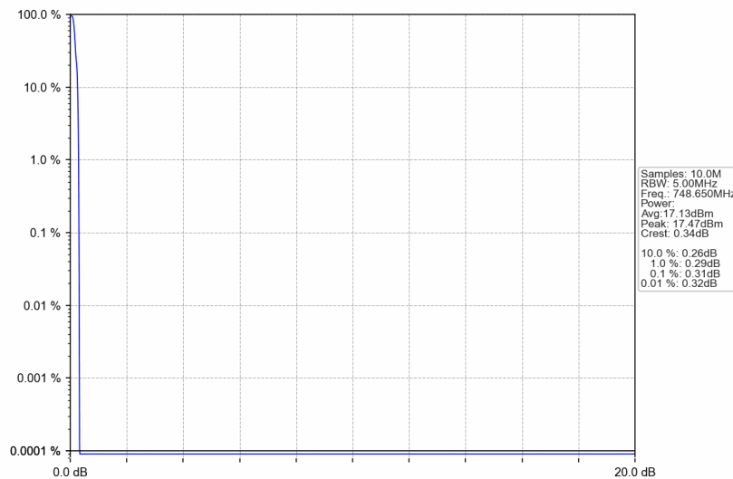
Band13_748.65MHz_GMSK_SISO_Ant1_NTNV_AGC+3
