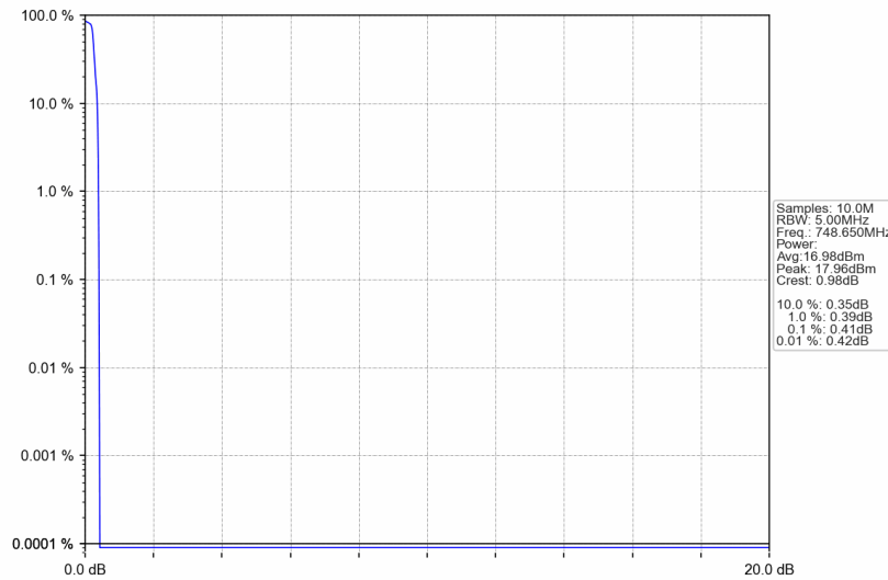
Band13_748.65MHz_GMSK_SISO_Ant1_NTNV_AGC
