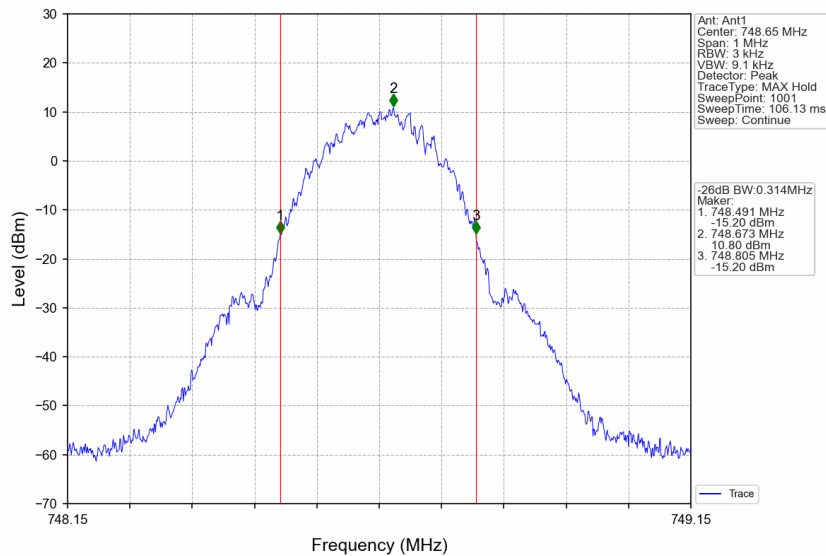
Band13_748.65MHz_GMSK_SISO_Ant1_NTNV_AGC+3
