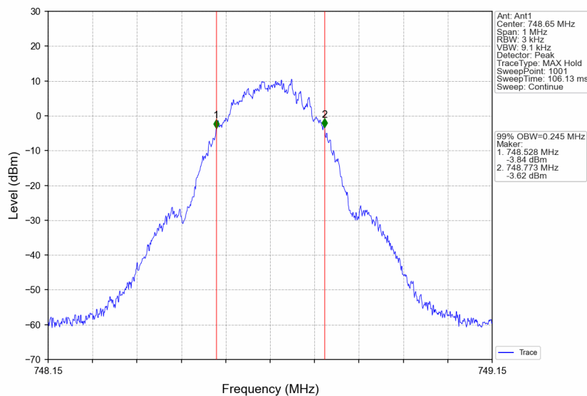
Band13_748.65MHz_GMSK_SISO_Ant1_NTNV_AGC+3
