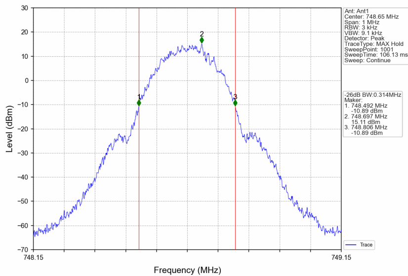
Band13_748.65MHz_GMSK_SISO_Ant1_NTNV_AGC
