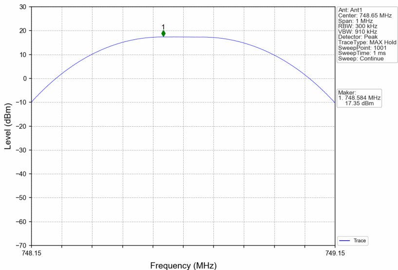
Band13_748.65MHz_GMSK_SISO_Ant1_NTNV_AGC+3
