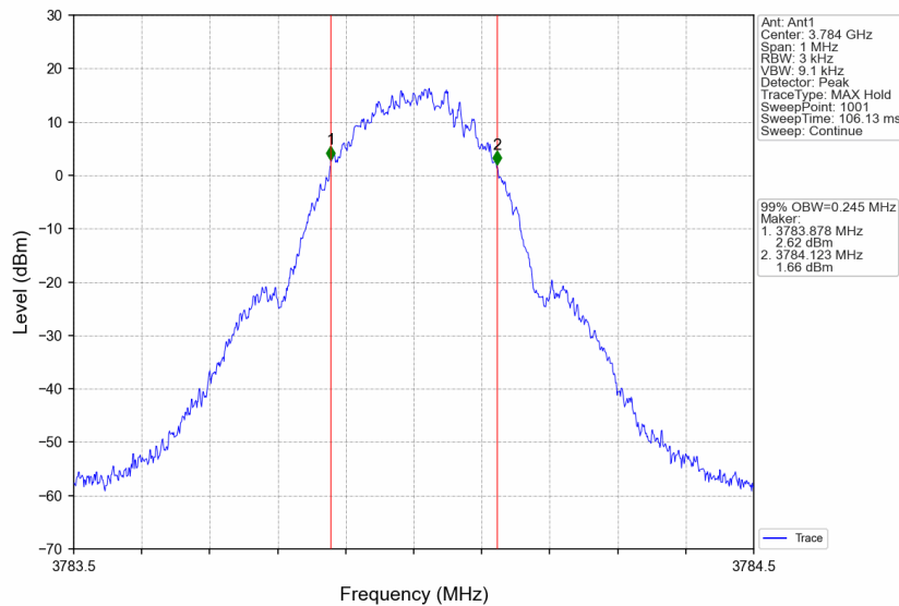
3780MHz-3980MHz_3784MHz_GMSK_SISO_Ant1_NTNV_AGC
