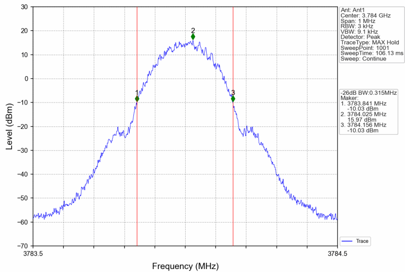
3780MHz-3980MHz_3784MHz_GMSK_SISO_Ant1_NTNV_AGC+3
