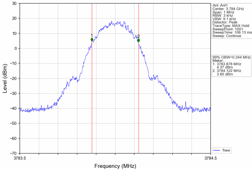
3780MHz-3980MHz_3784MHz_GMSK_SISO_Ant1_NTNV_AGC+3
