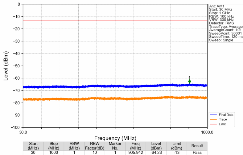
3780MHz-3980MHz_3979.9MHz_GMSK_SISO_Ant1_NTNV
