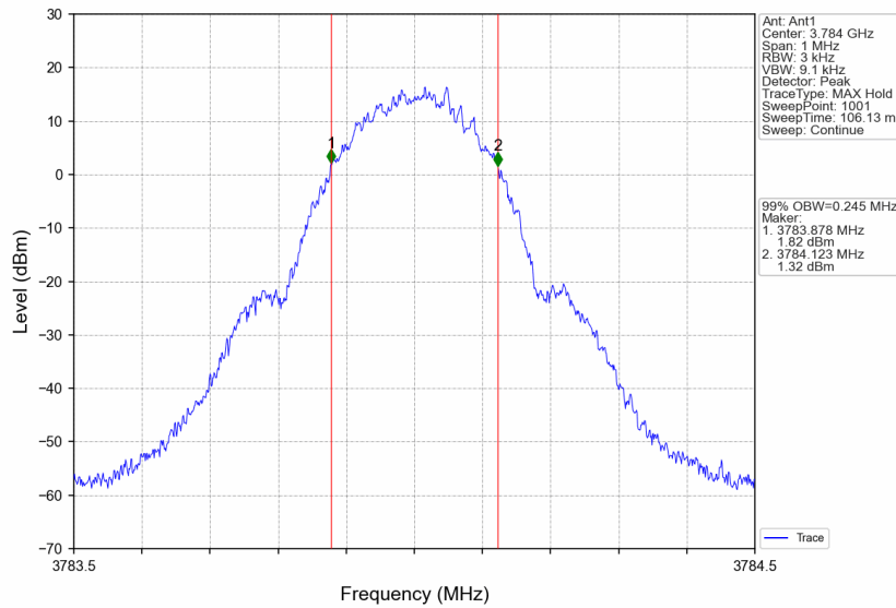
3780MHz-3980MHz_3784MHz_GMSK_SISO_Ant1_NTNV_AGC
