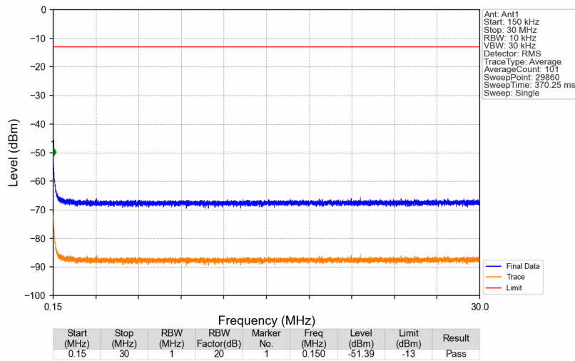
3780MHz-3980MHz_3780.1MHz_GMSK_SISO_Ant1_NTNV
