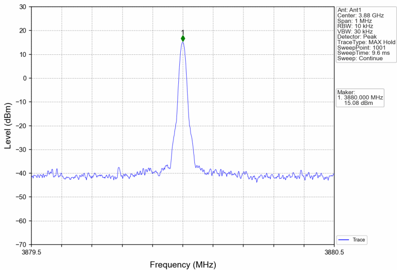
3780MHz-3980MHz_3880MHz_CW_SISO_Ant1_NTNV
