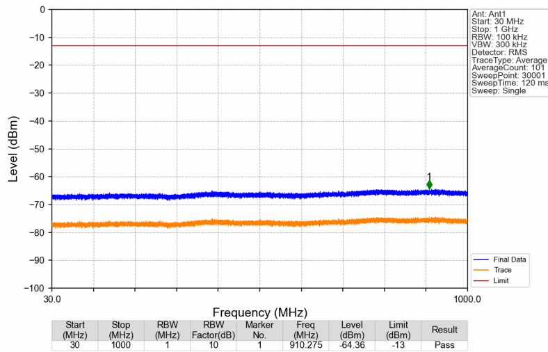
3780MHz-3980MHz_3780.1MHz_GMSK_SISO_Ant1_NTNV
