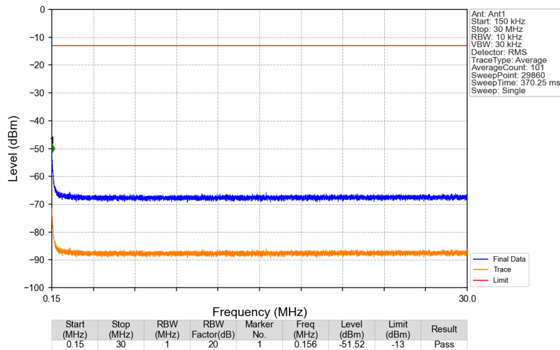
3780MHz-3980MHz_3979.9MHz_GMSK_SISO_Ant1_NTNV
