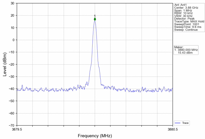
3780MHz-3980MHz_3880MHz_CW_SISO_Ant1_NTNV
