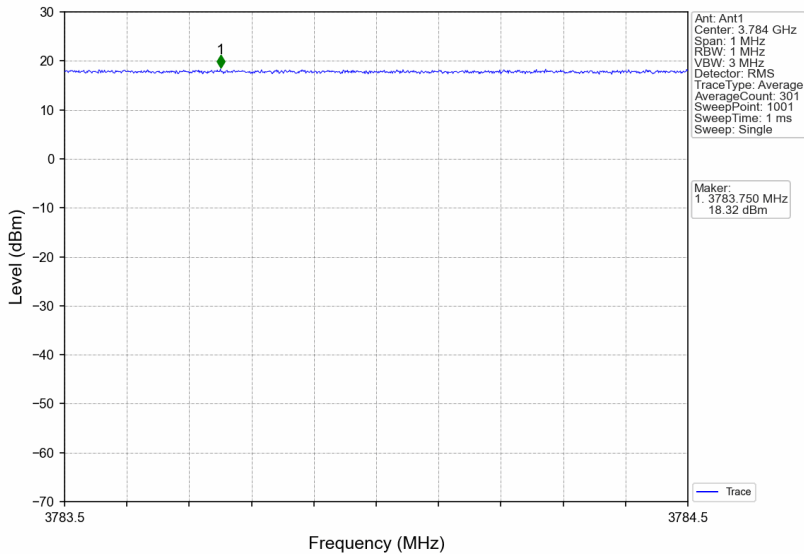
3780MHz-3980MHz_3784MHz_GMSK_SISO_Ant1_NTNV_AGC+3
